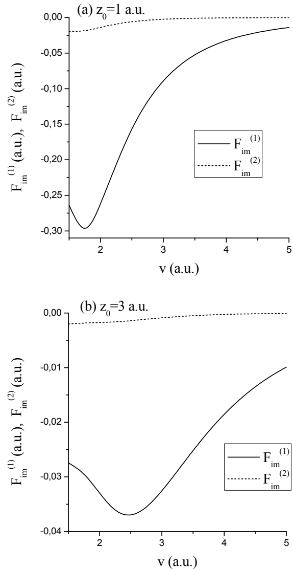
Слика 3. Зависност линеарне силе lika F_{im}^{(1)} и корекције F_{im}^{(2)} од брзине протона v , за два различита растојања од површине графена: (a) z_0 = 1 \text{ a.u.} и (b) z_0 = 3 \text{ a.u.} Figure 3. The linear image force F_{im}^{(1)} and the correction F_{im}^{(2)} versus the proton velocity v , for two positions: (a) z_0 = 1 \text{ a.u.} and (b) z_0 = 3 \text{ a.u.}
