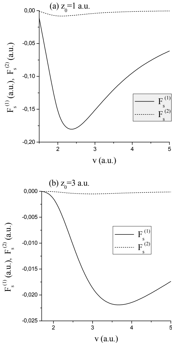
Слика 2. Зависност линеарне зауставне силе F_s^{(1)} и корекције F_s^{(2)} од брзине протона v , за два различита растојања од површине графена: (a) z_0 = 1 \text{ a.u.} и (b) z_0 = 3 \text{ a.u.} Figure 2. The linear stopping force F_s^{(1)} and the correction F_s^{(2)} versus the proton velocity v , for two positions: (a) z_0 = 1 \text{ a.u.} and (b) z_0 = 3 \text{ a.u.}
