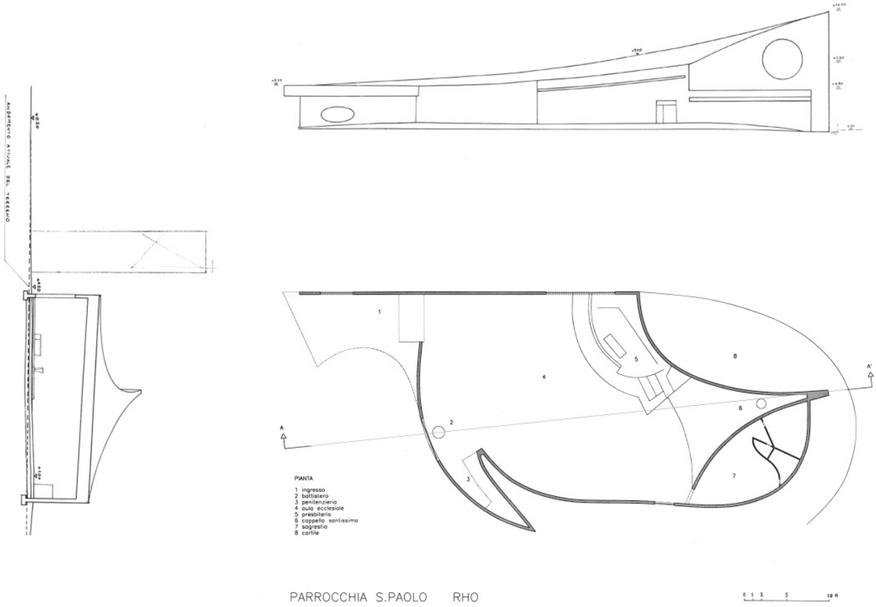
04 Maqueta en bronce de la propuesta definitiva. 05 Planta, alzado y secciones de la nueva iglesia.
