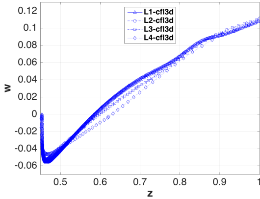
(d) CFL3D
