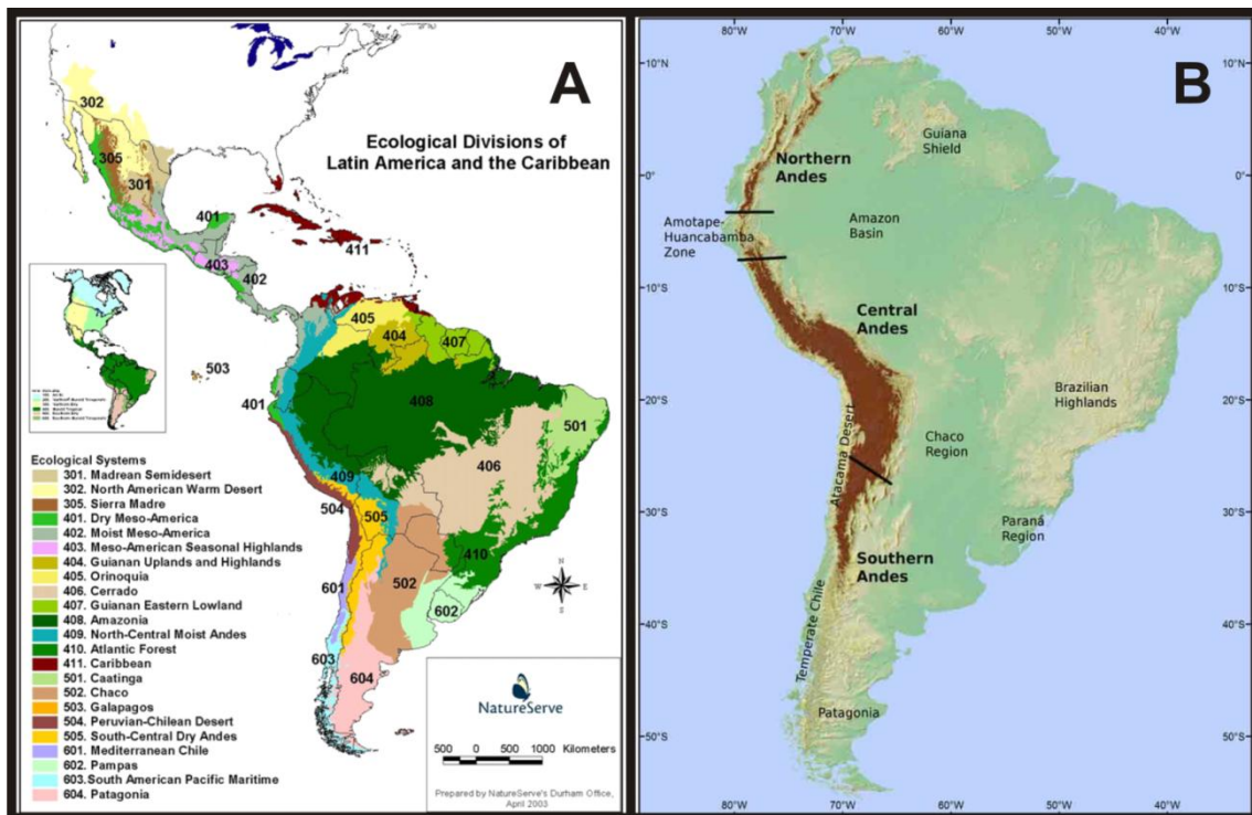
Figura 36. Mapas mostrando las áreas utilizadas para el análisis biogeográfico de Kaunia . A. Tomada de Josse et al., 2003. B. Tomada de Lueber y Weigend, 2014.
