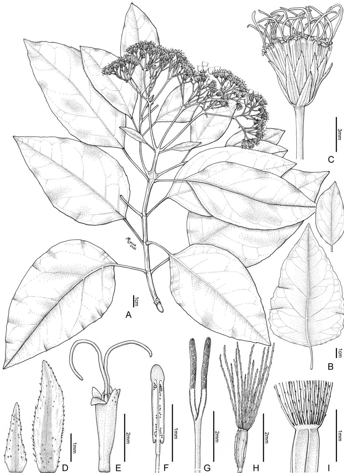
Figura 46. Kaunia gynoxymorpha . A, Rama con inflorescencia secundaria. B, Variación del margen y forma de la lámina. C, Capítulo. D, Filarios, externo a la izquierda, interno a la derecha. E, Flor sin cipsela ni papus. F, Estambre. G, Estilo. H, Cipsela y papus. I, Detalle de anillo formado por base de cerdas del papus (A-I: Nee y Bohls 49760, F).
