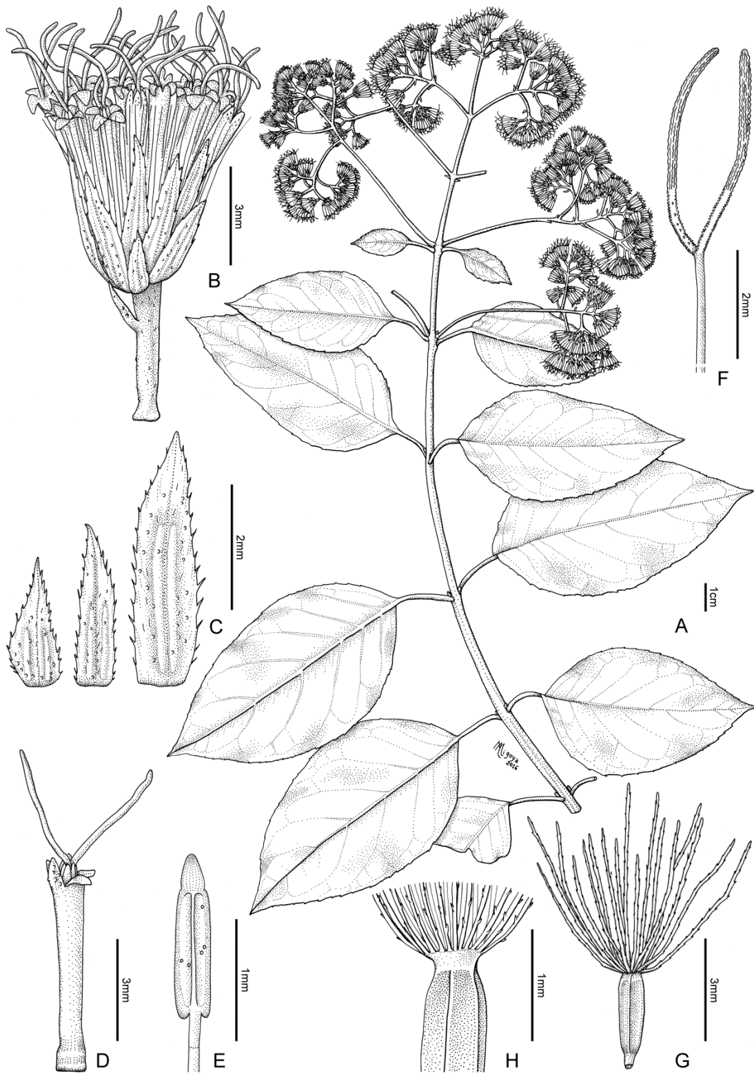
Figura 42. Kaunia endyta . A, Rama con inflorescencia secundaria. B, Capítulo. C, Filarios, más externos a más internos de izquierda a derecha. D, Flor sin cipsela ni papis. E, Estambre. F, Estilo. G, Cipsela y papus. H, Detalle de anillo formado por base de cerdas del papus (A-H: Beck 32690, LP).
