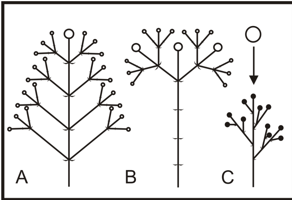
Figura 6. Tipos de capitulescencias encontradas en Kaunia . A, Tirsoide. B, Cimoide. C, Detalle de paraclados de cuarto orden. Los círculos negros corresponden a los capítulos; los círculos blancos corresponden a la estructura representada en C.
