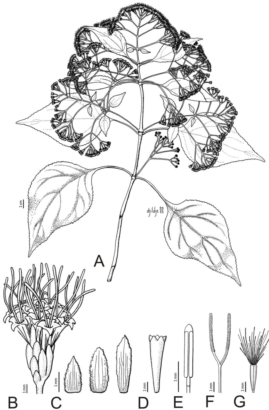
Figura 52. Kaunia lasiophthalma . A, Rama con inflorescencia secundaria. B, Capítulo. C, Filarios, externos a internos de izquierda a derecha. D, Corola. E, Estambre. F, Estilo. G, Cipsela y pappus (A-G: Meyer, T. 4307, LP).
