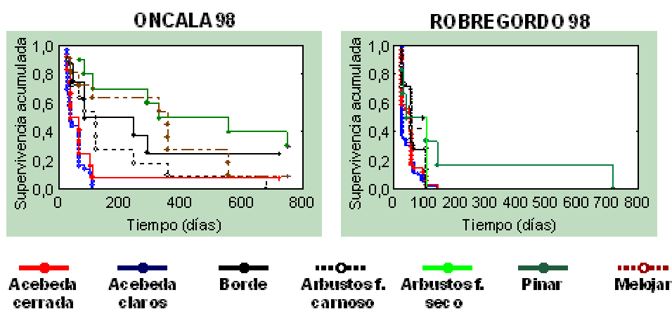
Figura 2. Curvas de supervivencia de las plántulas en los distintos microhábitats, y en ambas acebedas.
