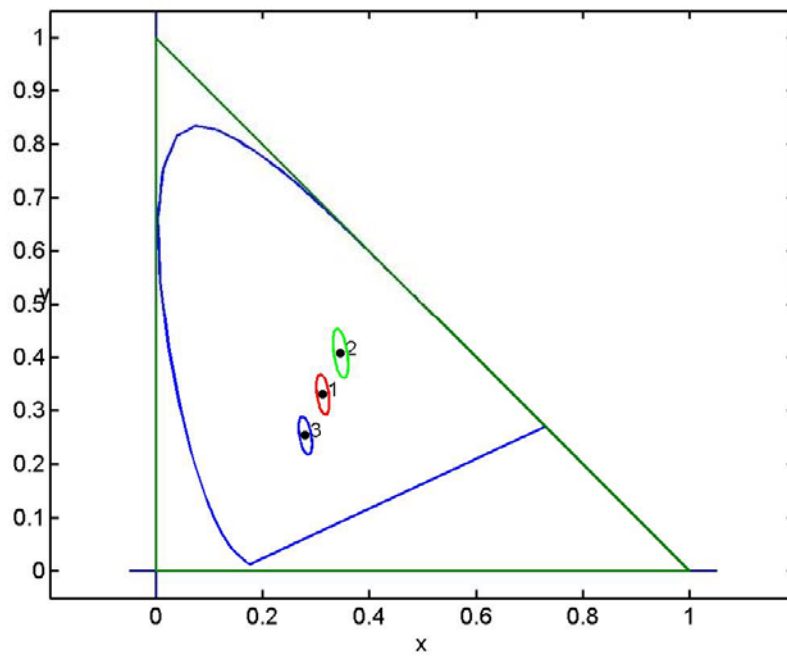
Figura 14: Elipse de MacAdam para el filtro Verde.
