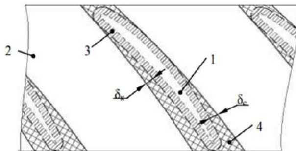
Рис. 9 - Погрешность формообразования межлопаточных каналов кольцевым инструментом: 1 – теоретический профиль пера лопатки; 2 – удаленный объем материала межлопаточного канала; 3 – слой притупка; 4 – слой металла, образованный из-за погрешности формообразования.
