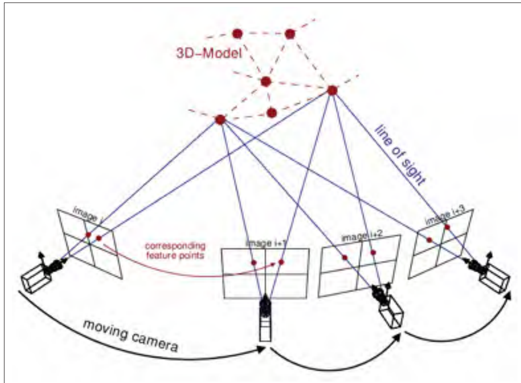
Figure 1.6 Principe des approches SFM Tirée de http://www.theia-sfm.org/sfm.html
