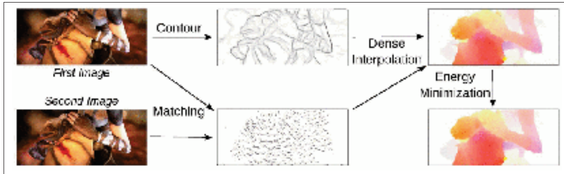
Figure 1.8 Étapes de l'EpicFlow Tirée de Revaud et al. (2015, p. 2)
