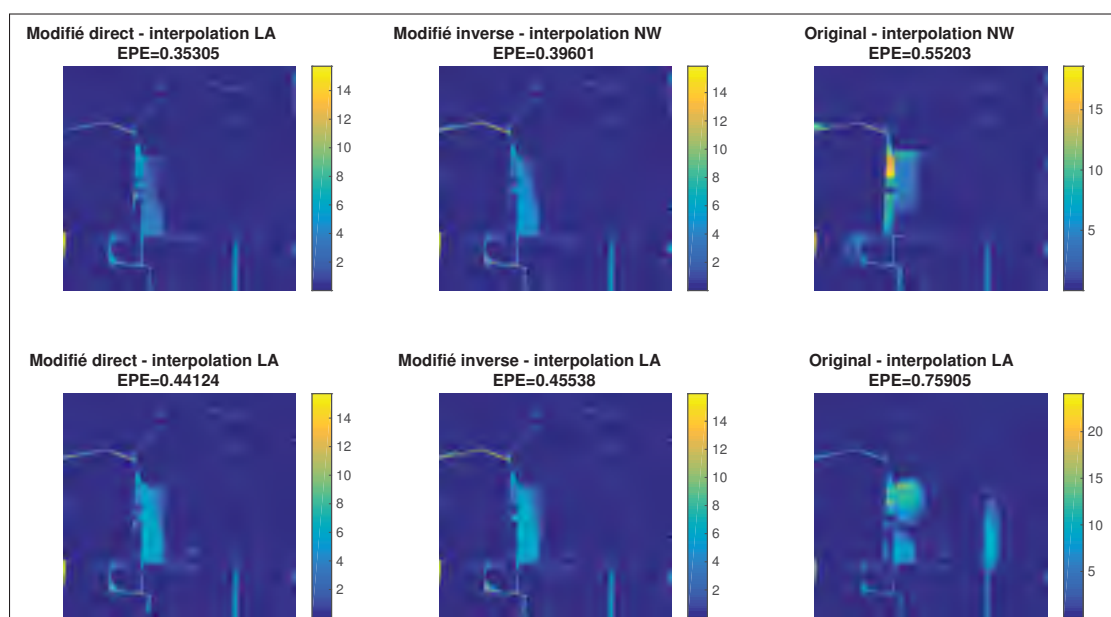
Figure 3.3 Répartition des erreurs EPE sur l'ensemble des pixels de l'image sur l'exemple Urban3 de Middlebury
