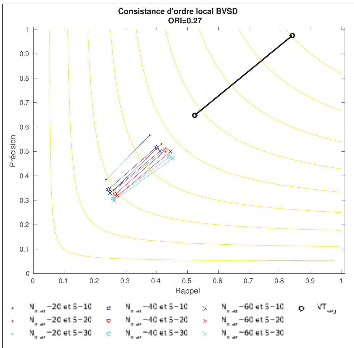
Figure 3.11 Consistance d'ordre locale des séquences de la base de données BVSD
