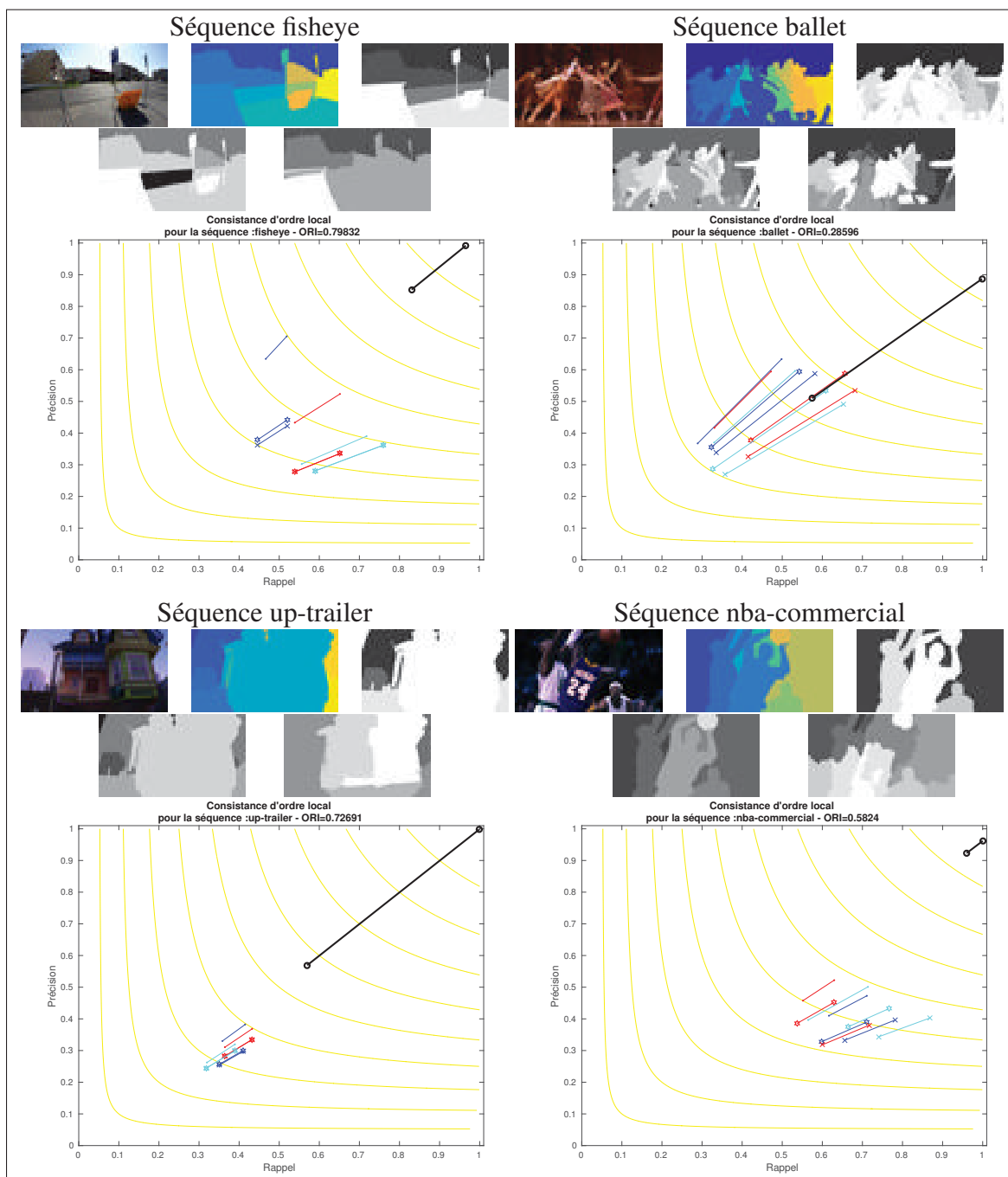
Figure 3.13 Consistance d'ordre local pour les séquences fisheye , up-trailer , ballet et nba-commercial de la BVSD Pour chaque séquence, de gauche à droite, de haut en bas est représenté : la séquence traitée, les vérités terrain de la segmentation et de l'ordre, l'ordre obtenu avec la vérité terrain de segmentation ainsi que l'ordre (celui de l'ORI)
