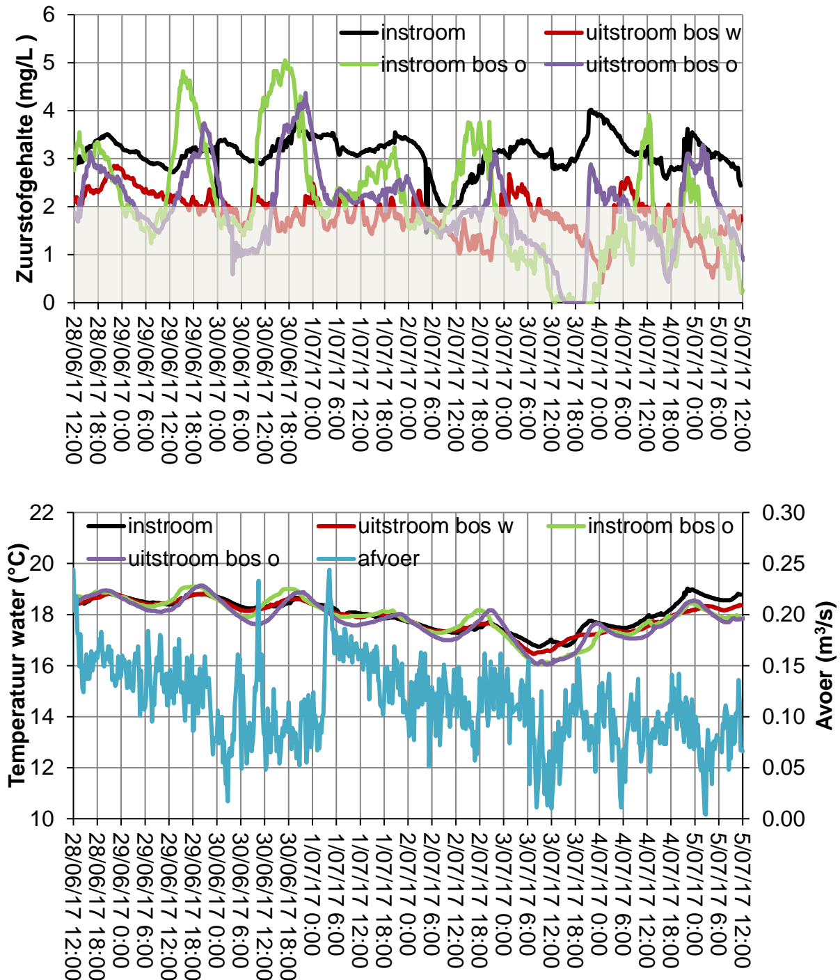
Figuur 12: Continuumetingen zuurstofgehalte (boven) en temperatuur en afvoer (onder) op vier plekken in het gebied. In de zuurstofgrafiek geeft de grijze balk de hypoxische zone aan. De inzet geeft de ligging van de meetpunten weer. Ligging locaties is aangegeven in figuur 11.
