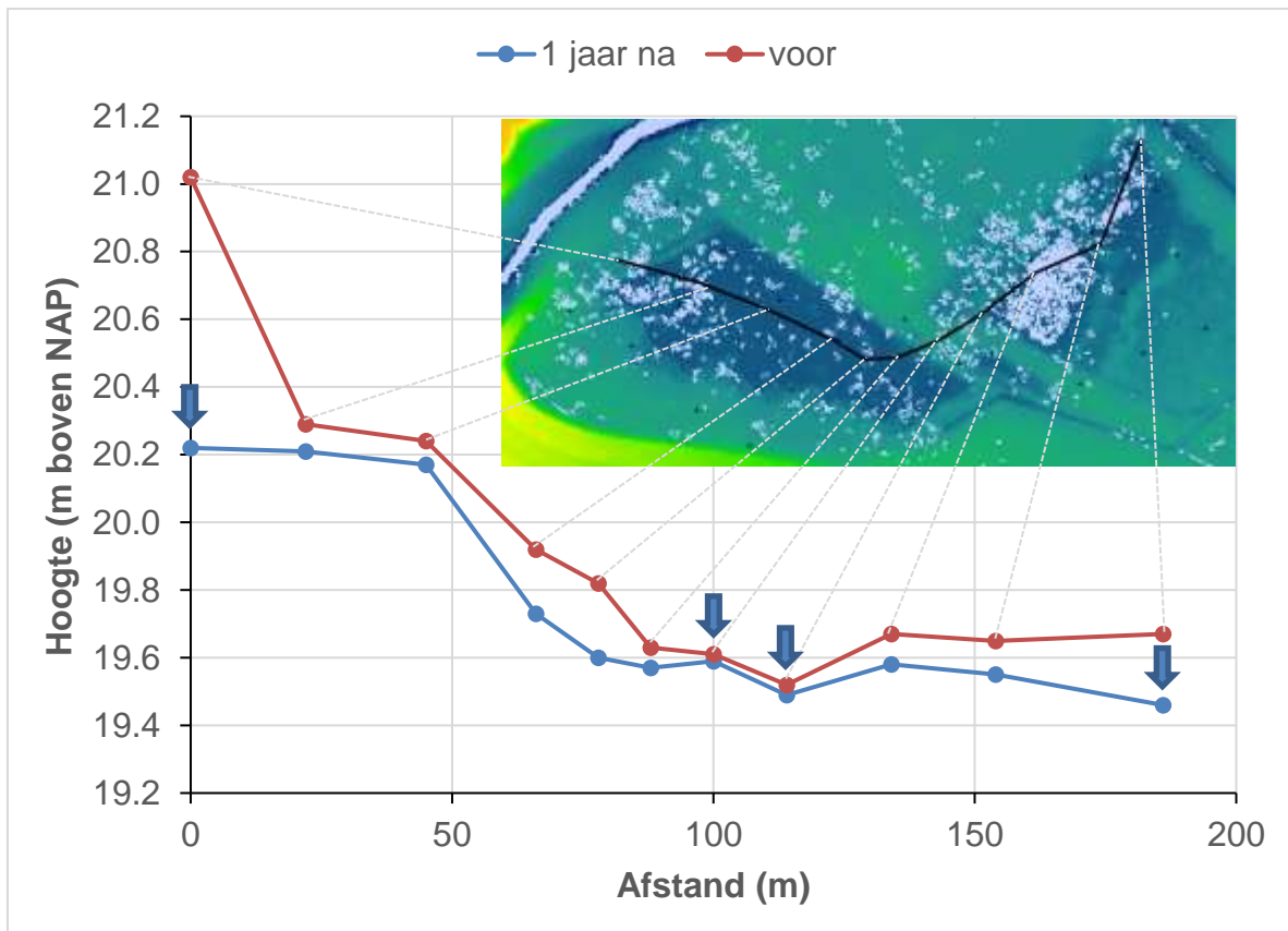
Figuur 7: Verandering in bodemhoogte op het laagste punt per transect vlak voor en 1 jaar na uitvoering. De posities aangegeven met pijlen zijn doorgraven tijdens uitvoering van de maatregel. De inzet geeft de ligging van de punten weer, onderling verbonden met zwarte lijn.
