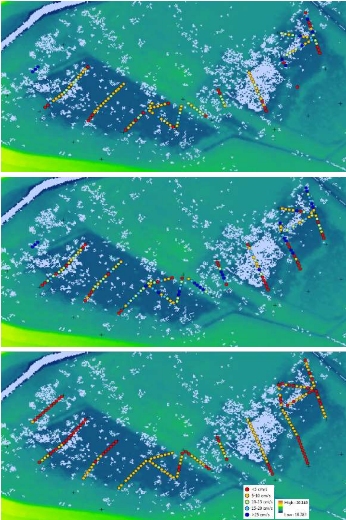
Figuur 6: Stroomsnelheden op 18 januari (ca. 0,2\text{ m}^3/\text{s} ), 9 maart (afvoerpiek, 2,7\text{ m}^3/\text{s} ) en september (beek afgedamd door bever) geprojecteerd op de hoogtekartaat (oorspronkelijke situatie; doorgravingen niet zichtbaar).
