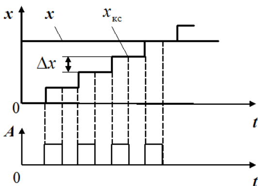
Рисунок 4.9 – ЦВП число-імпульсного квантування
