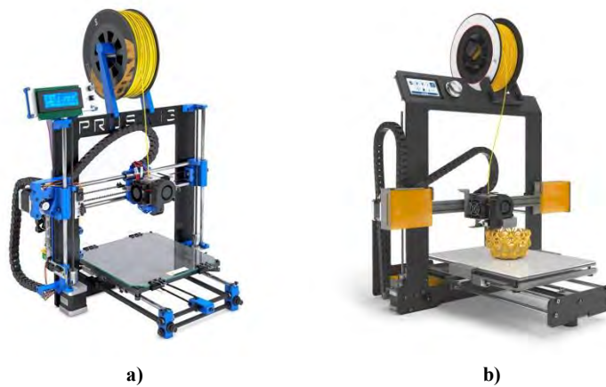
Figura 1: Impresoras 3D disponibles en el Fab Lab ETSIDI a) Prusa i3 Hephestos y b) Hephestos 2.
