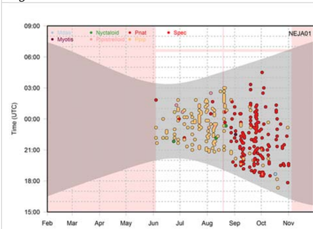
Figure 3.21 Neeltje Jans 2015
