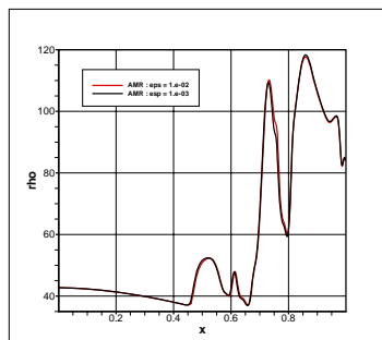
Figure 5– Tube à choc : Variation le long de la paroi basse de la masse volumique à un temps t=1 , pour deux valeurs du paramètre de raffinement \varepsilon=10^{-2} et 10^{-3} .
