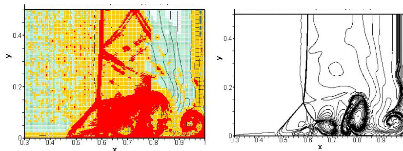
Figure 4– Tube à choc ( Re=200 ) : maillage adaptatif (à gauche) et iso-contours de masse volumique (à droite), pour la valeur du paramètre de raffinement \varepsilon=10^{-2} et à t=1 .
