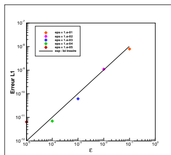
Figure 3– Évaluation de l'erreur d'approximation en fonction du paramètre de raffinement \varepsilon .
