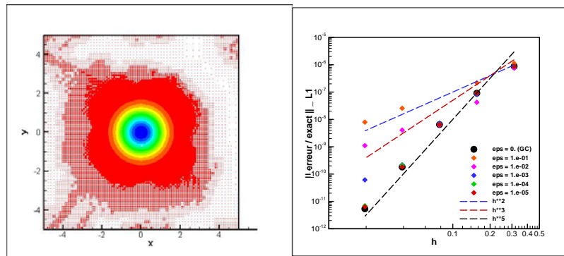
Figure 1– Convection d'un tourbillon : solution à t=10 , valeur de la masse volumique sur le maillage adapté pour \varepsilon=10^{-2} à partir d'un maillage 512 \times 512 (à gauche) et taux de convergence et influence du processus de multirésolution (à droite).
