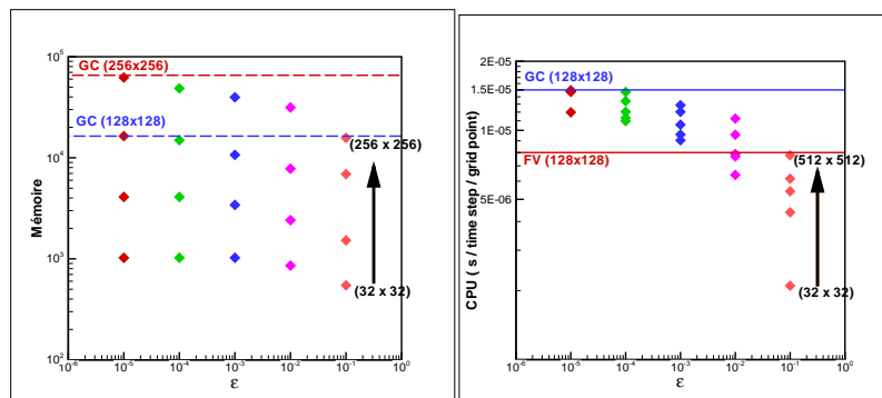
Figure 2– Convection d'un tourbillon : Efficacité de la méthode de multirésolution sur la mémoire (à gauche) et le CPU (à droite) en fonction du seuil ( \varepsilon ).
