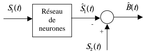
FIG. 2 : Schéma de fonctionnement
