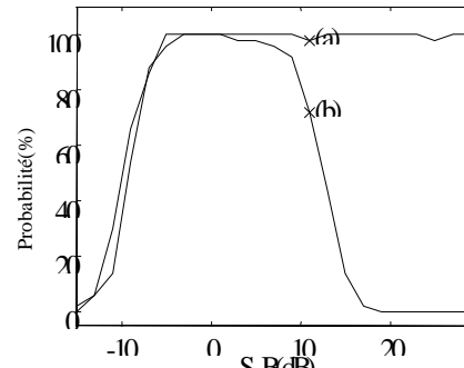
Figure 5 : Détection cyclique \alpha=2\text{Mhz} \tau=0,25\mu\text{s} \epsilon=-1 (a) après focalisation (b) avant focalisation
