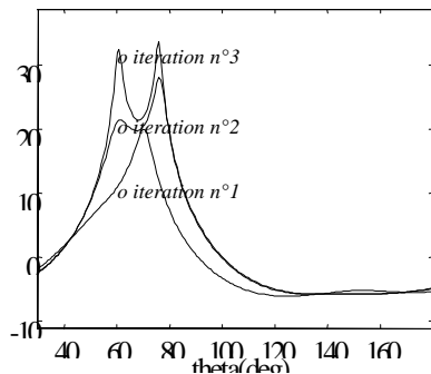
Figure 2 : Focalisation cyclique : \alpha=2\text{Mhz} \tau=0,25\mu\text{s} \epsilon=-1
