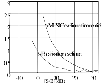
Figure 4 : MUSIC cyclique : \alpha=1,5\text{Mhz} \tau=0,33\mu\text{s} \epsilon=-1
