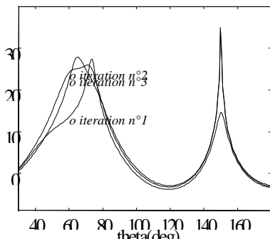
Figure 3 : Focalisation classique : \alpha=0 \tau=0 \epsilon=-1
