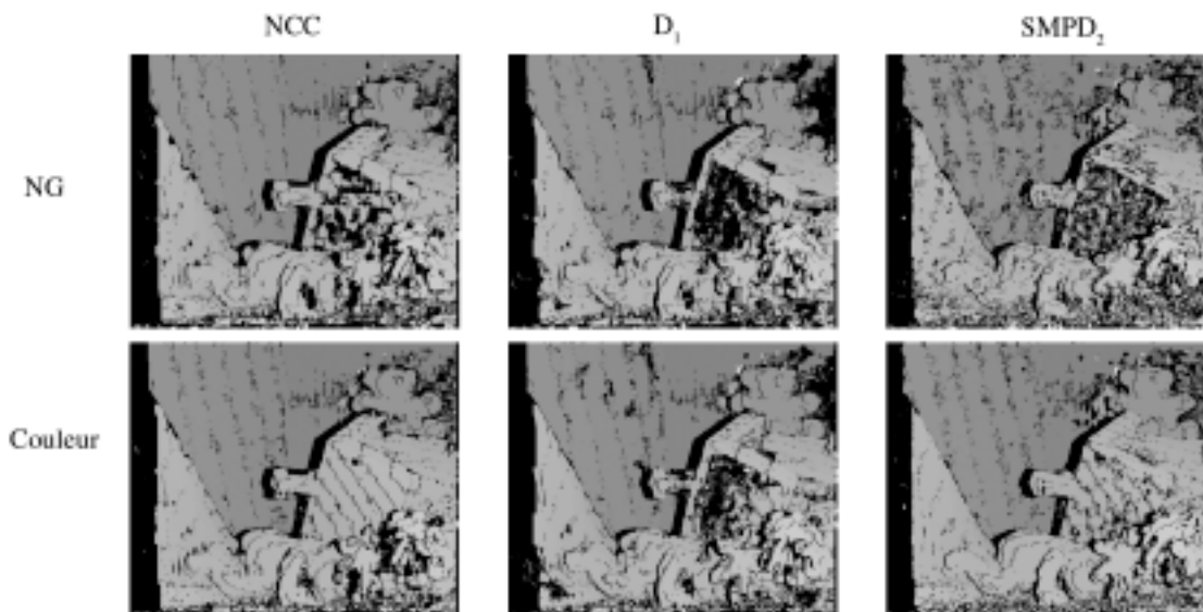
Figure 12. Teddy : comparaison des cartes de disparités obtenues avec les images couleur et les images de niveaux de gris pour deux mesures classiques et une mesure robuste.
