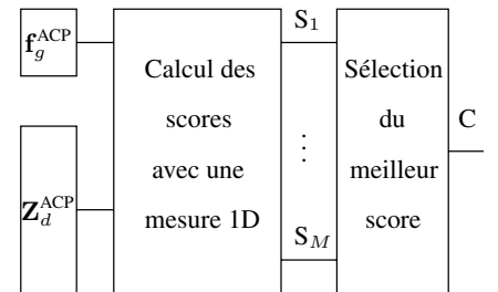
Figure 4. MÉTHODE ACP-IMAGE ( S = Score , C = Correspondant , voir figure 1(c) pour le calcul des scores avec une mesure 1D).
