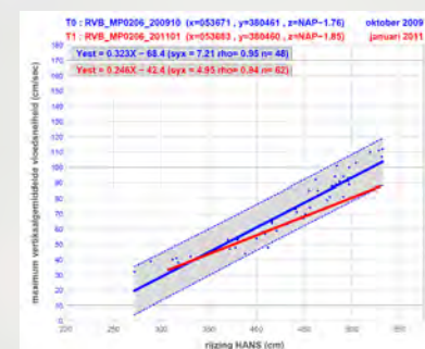
Figuur 3: Maximale vloednelheid i.f.v. rijzing (meting Rug van Baarland – raai 2 – punt t.h.v. LW-lijn)
