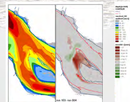
Figuur 2: Maximale vloednelheid (numeriek model)
