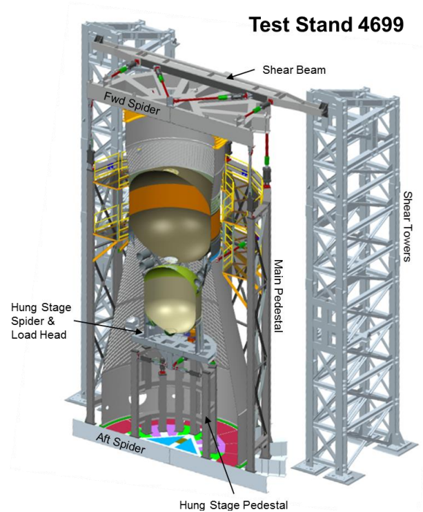
Figure 10 Arrangement of test articles for the IST
