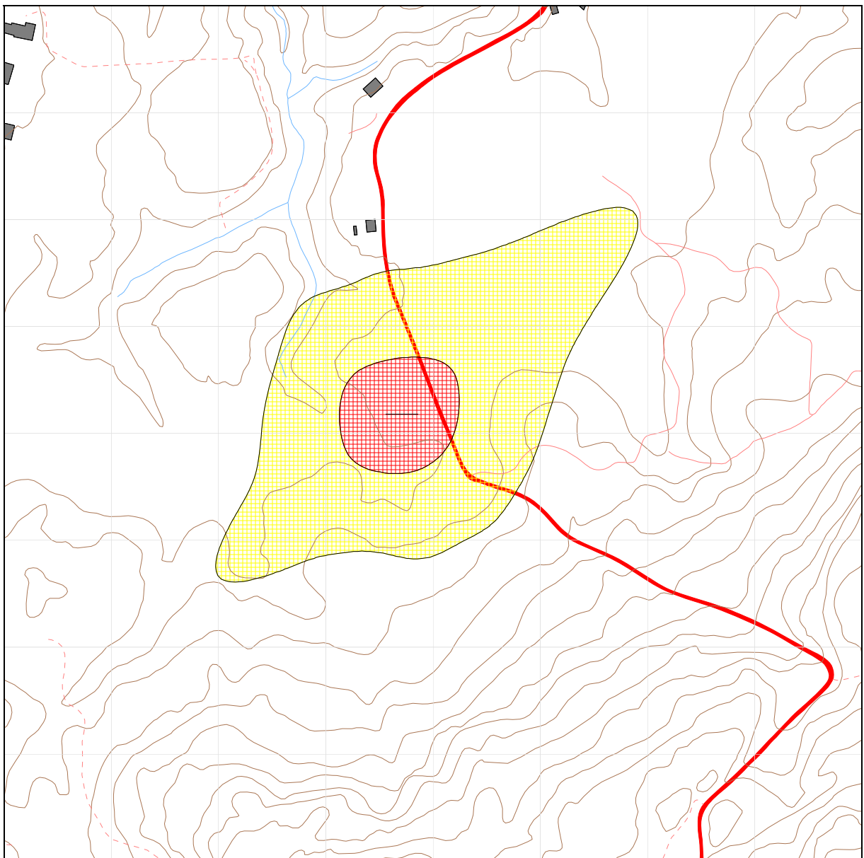
Figur 5-1 Støysoner for den planlagte Orderud helikopterplass, Trøgstad. M 1:5 000.
