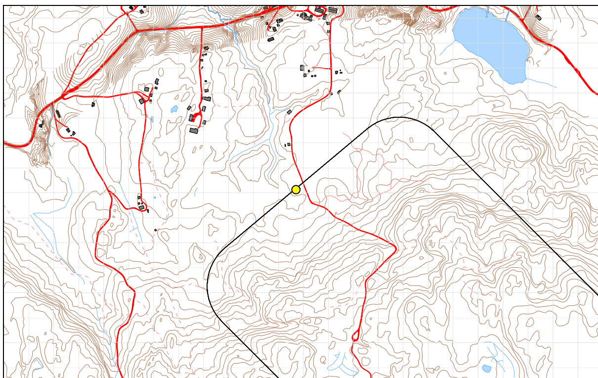
Figur 4-1 Landingsplassen markert med gul sirkel og hoved inn- og utflygingsretninger. M 1:15 000.
