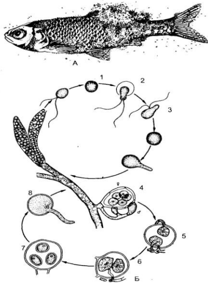
Рис. 1. Життєвий цикл сапролегнії паразитичної Saprolegnia parasitica
