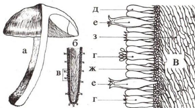
Рис.14. Розріз плодового тіла та фрагмент трами та гіменію у шапінкових грибів
