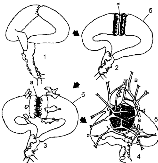
Рис. 4. Розвиток зигоспор при зигогамії у фікоміцеса Phycomyces blakesleeanus
