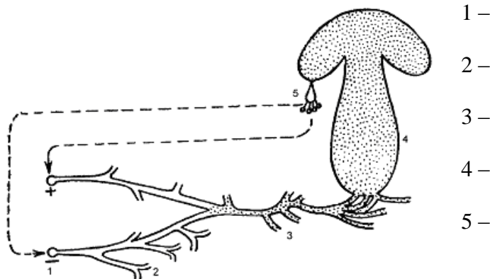
Рис.13. Цикл розвитку шапінкового гриба
