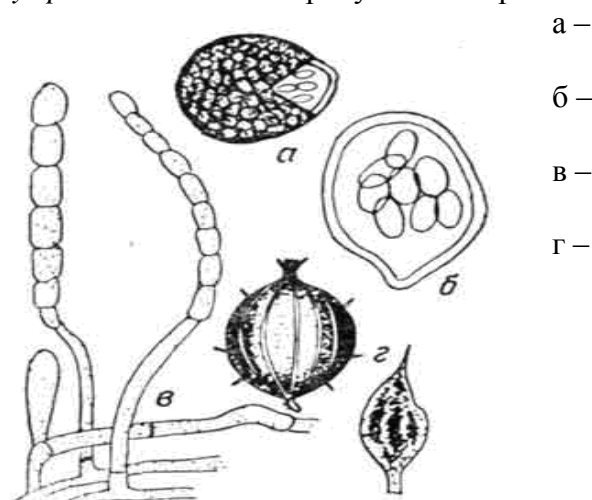
Рис.9. Сферотека агрусова Podosphaera mors-uvae
