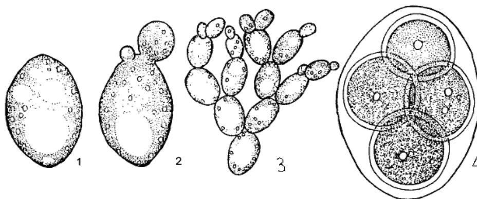
Рис. 7. Цукрові дріжджі Saccharomyces cerevisiae
