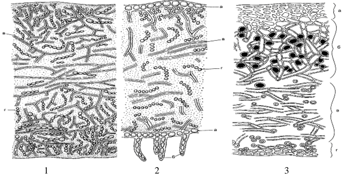
Рис. 19. Анатомічна будова слані лишайників: 1 – Collema , 2 – Leptogium , 3 – Xanthoria
