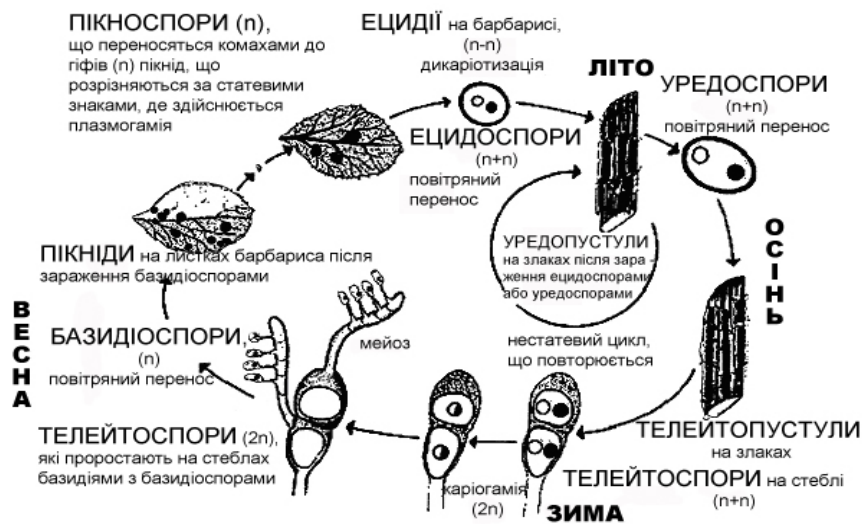
Рис. 17. Цикл розвитку іржі злаків Puccinia graminis
