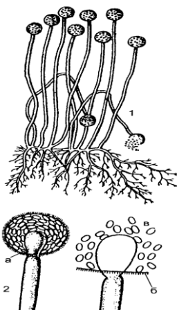
Рис. 5. Міцелій та органи розмноження мукора Mucor
