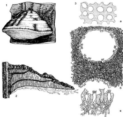
Рис. 12. Трутовик справжній Fomes fomentarius
