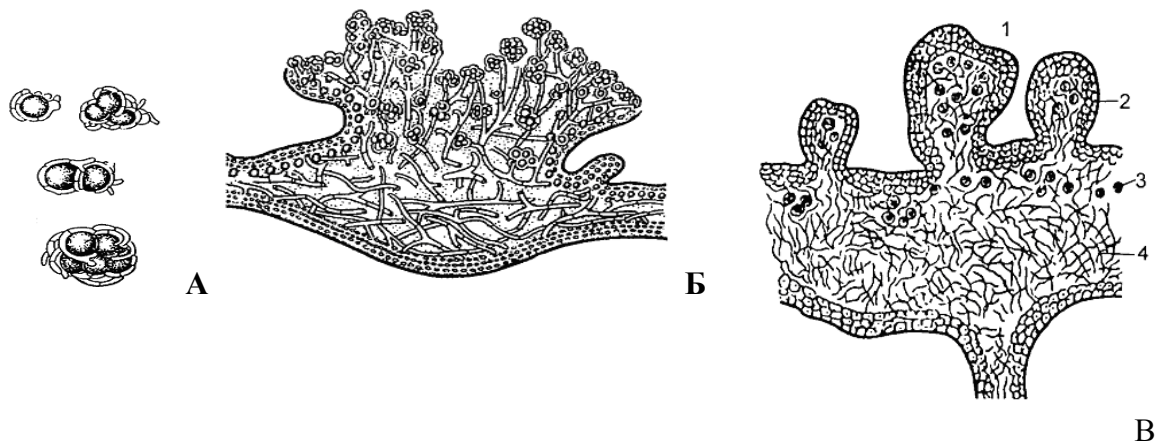
Рис.20. Органи вегетативного розмноження лишайників
