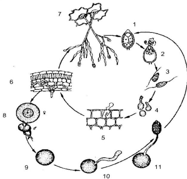
Рис. 3. Життєвий цикл фітофтори інфекційної Phytophthora infestans
