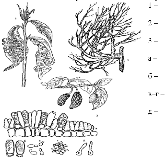
Рис.8. Тафринові гриби з роду Taphrina
