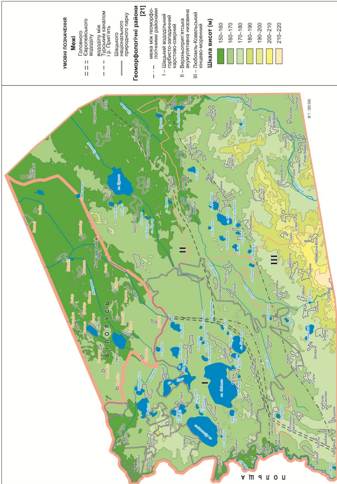
Рис. 3.6. Сучасний рельєф (склала О. В. Антишок)
