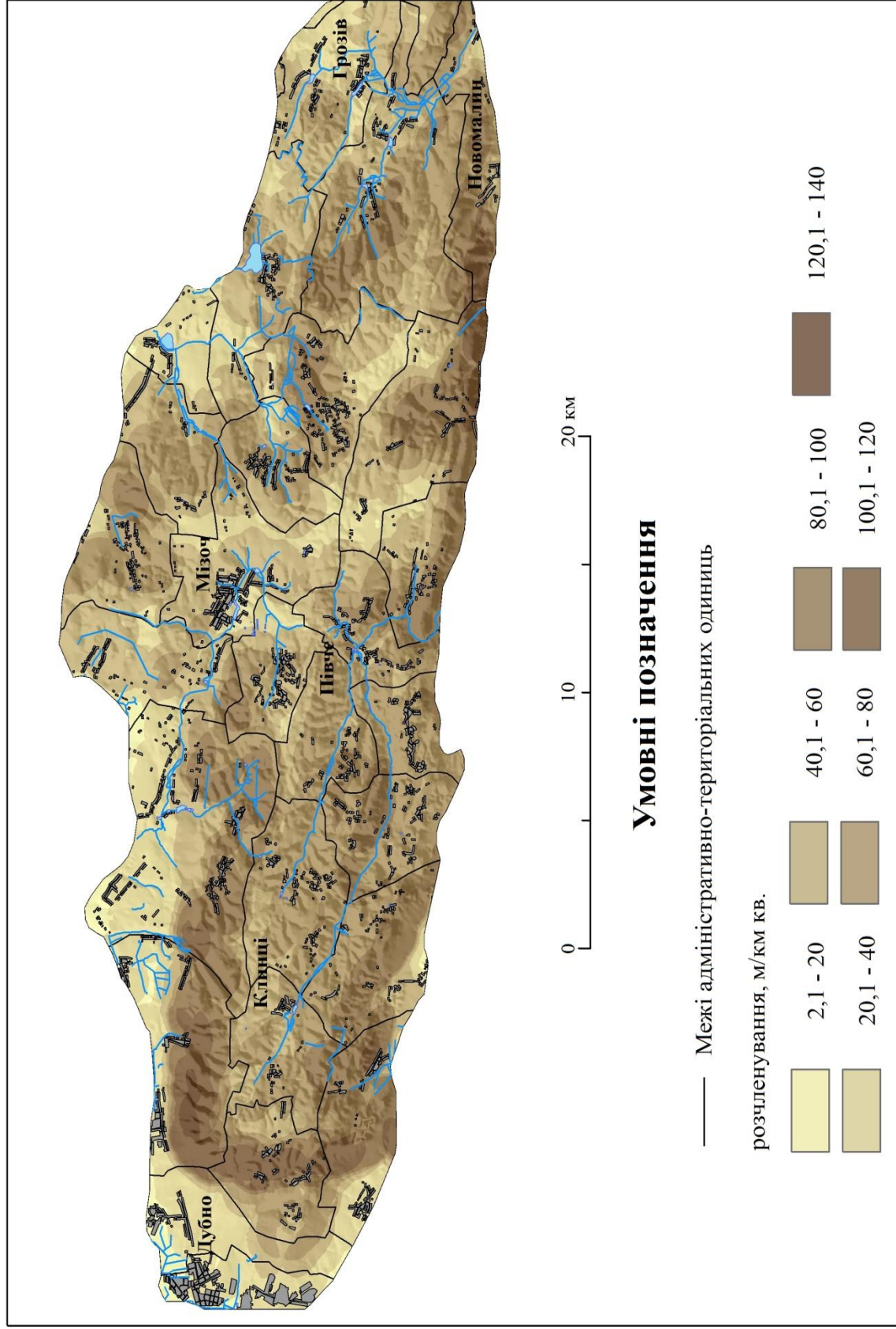
Рис. 3. Розподіл показника вертикального розчленування рельєфу Мізоцького краю
