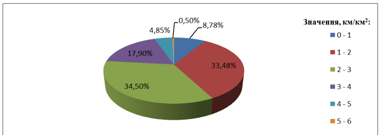
Рис. 4. Розподіл значень горизонтального розчленування рельєфу Мізоцького кряжу
