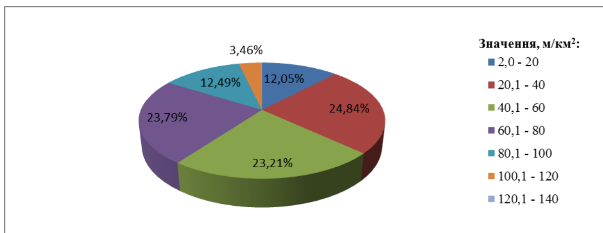
Рисунок 2. Розподіл значень вертикального розчленування рельєфу Мізоцького кряжу
