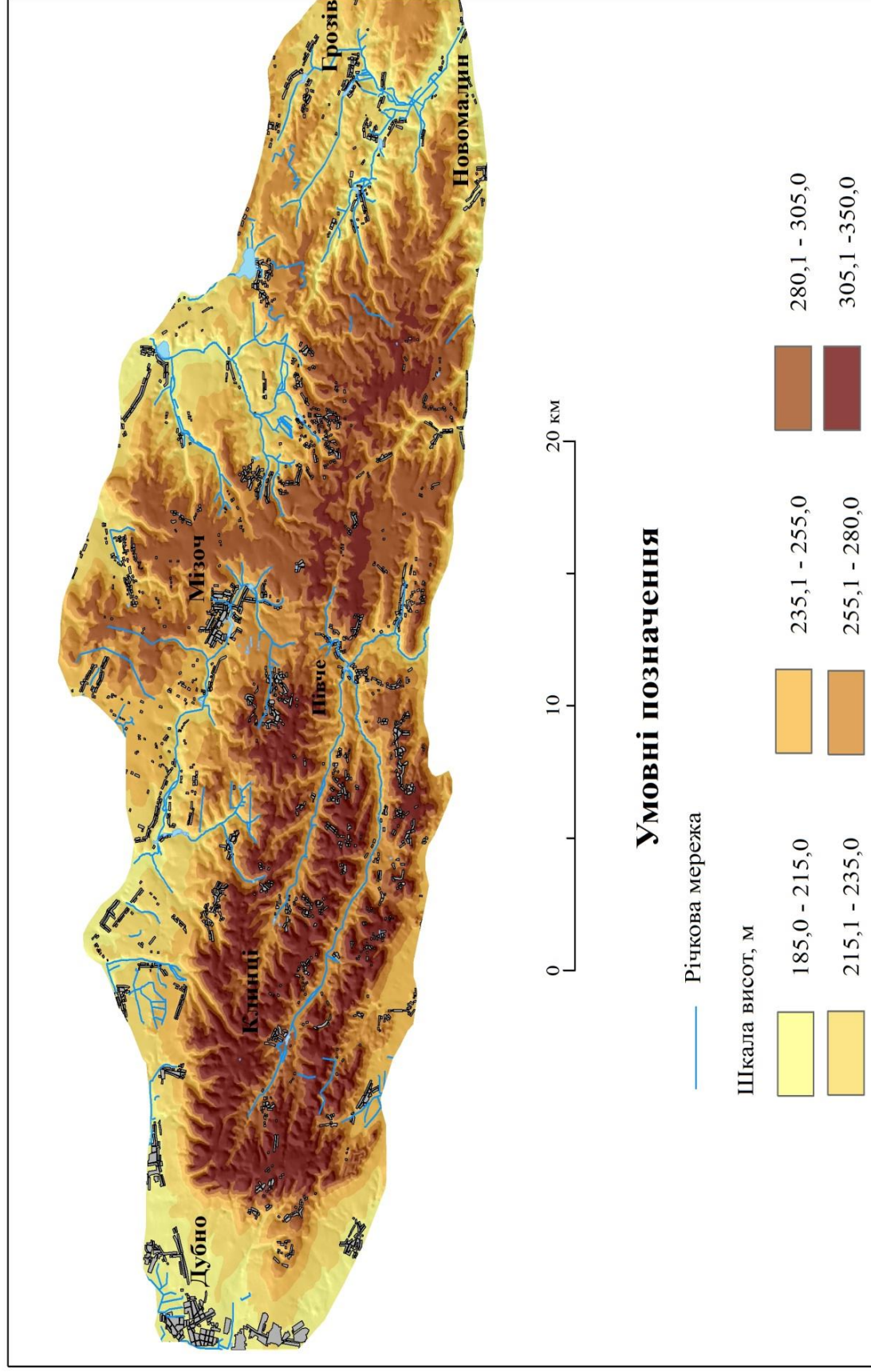
Рис. 1. Цифрова модель рельєфу Мізоцького краю
