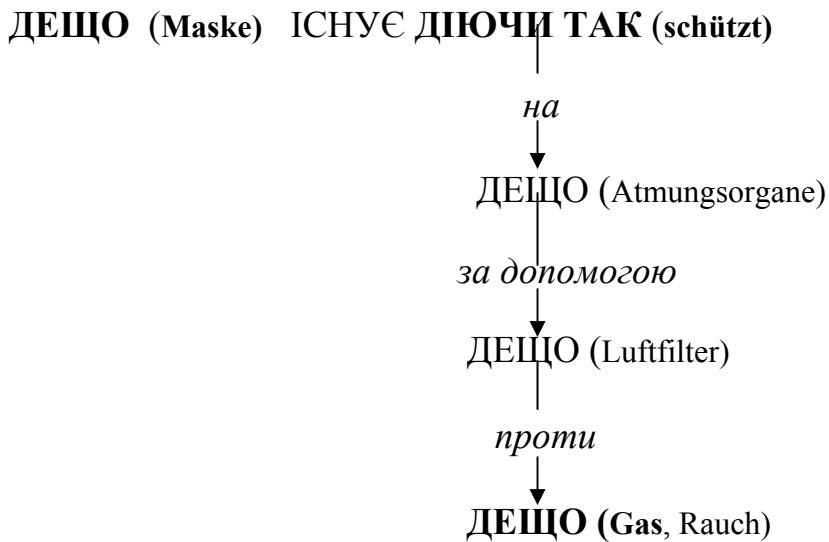
Рис. 1. Фрейм GASMASKE
