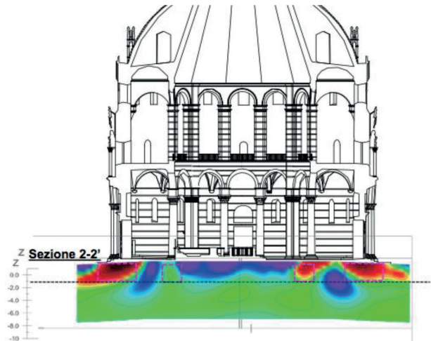
Fig. 17 – Results of ERT for Baptistry. Fig. 17 – Risultati delle tomografie elettriche sul Battistero di Piazza Duomo. Si noti la “presenza” della fondazione anche sul lato esterno.
