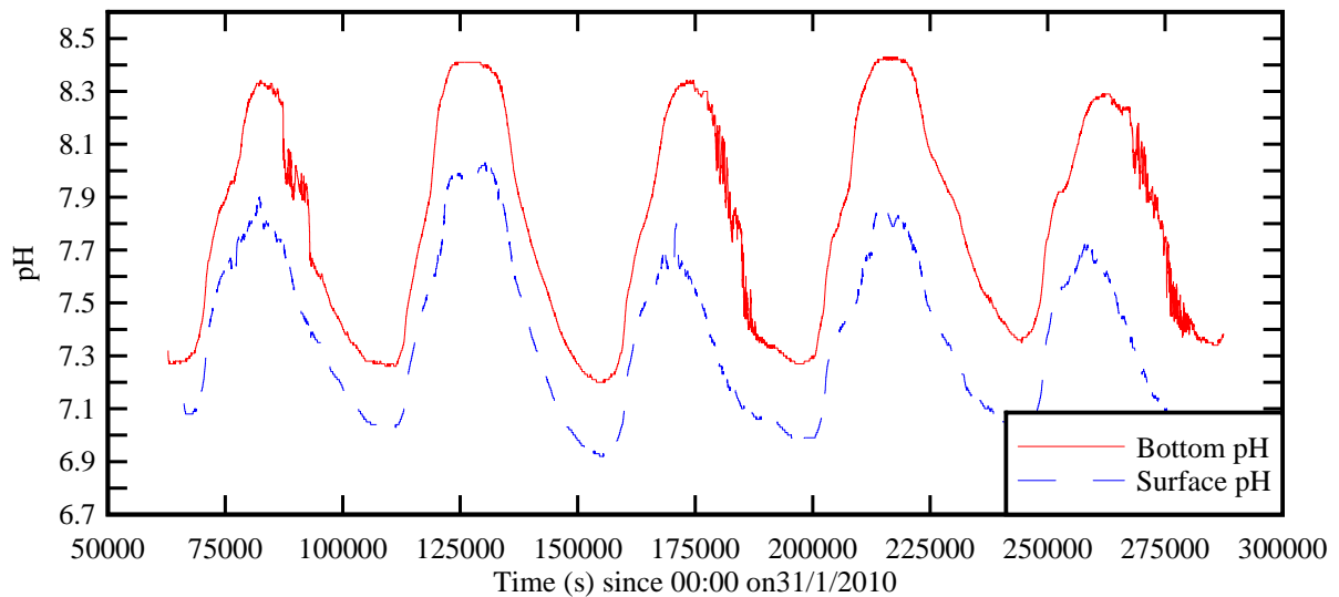
(D) pH at Site 2B
