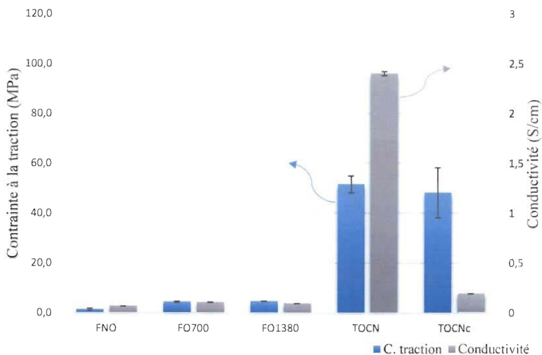
Figure 6.6 Conductivité électrique et tenue mécanique des différents composites
