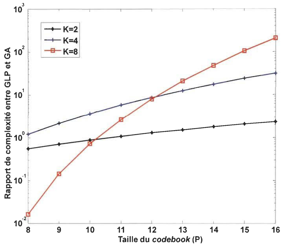
Figure 4.13. Rapport de complexité entre le précodage à base de GA et la méthode de Fang et al. [50] en fonction de la taille du codebook .
