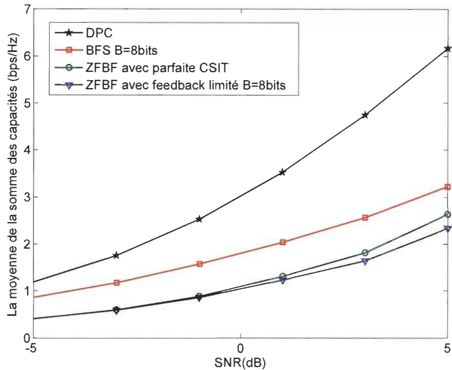
Figure 5.6. Comparaison de la moyenne de la somme des capacités entre le DPC, le BFS, le ZFBF avec parfaite CSIT et feedback limité [8] pour un système MU-MIMO avec K = 3 , N_t = 3 , N_r = 1 et B = 8 bits.
