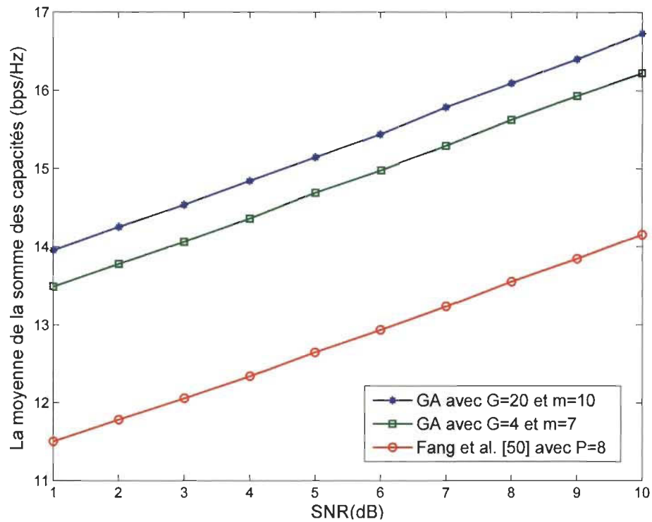
Figure 4.11. Comparaison de la moyenne de la somme des capacités entre le précodage à base de GA et la méthode de Fang et al. [50] pour un système MU-MIMO avec K = 2 , N_t = 2 et N_r = 2
