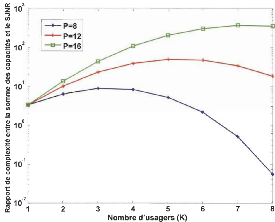
Figure 4.6. Rapport de complexité entre le critère de la maximisation du SJNR et le critère de Fang et al. [50] en fonction du nombre d'utilisateurs.
