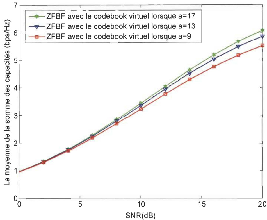
Figure 3.9. Comparaison en termes de moyenne de la somme des capacités entre codebooks virtuels conçus avec différentes longueurs de a pour un système MU-MIMO avec N_t = 2 , b = 2 et B = 4 bits.
