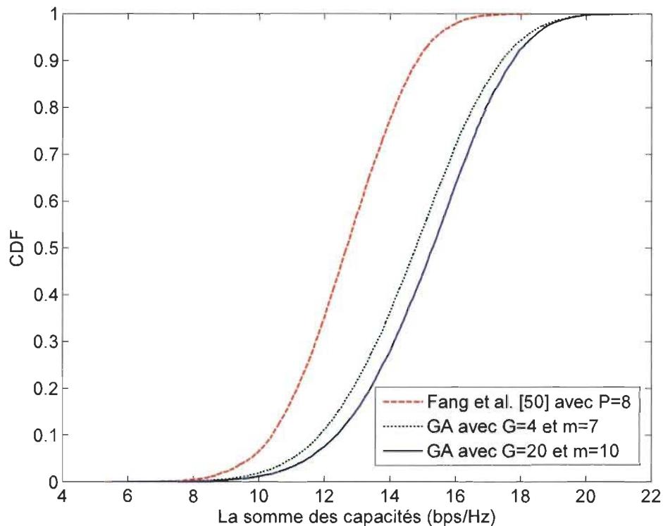
Figure 4.10. Comparaison de la CDF de la somme des capacités entre le précodage à base de GA et la méthode de Fang et al. [50] pour un système MU-MIMO avec K = 2 , N_t = 2 et N_r = 2 .
