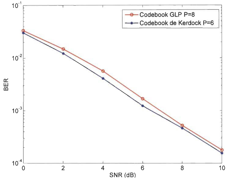
Figure 3.5. Performance en BER pour le précodage à base des codebooks GLP et de Kerdock pour un système MU-MIMO avec feedback limité pour X = 10 , K = 2 , N_t = 2 et N_r = 2 .
