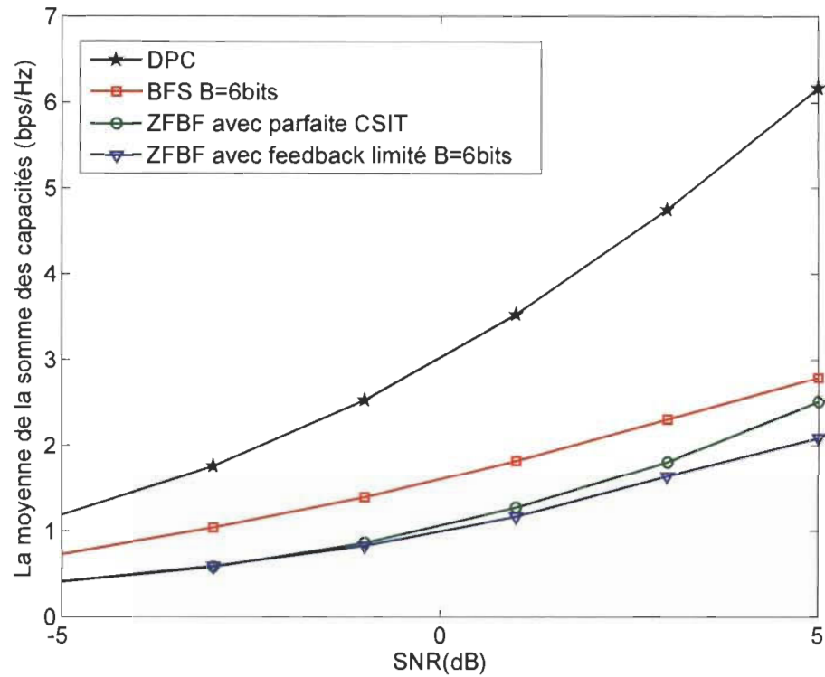
Figure 5.7. Comparaison de la moyenne de la somme des capacités entre le DPC, le BFS, le ZFBF avec parfaite CSIT et feedback limité [8] pour un système MU-MIMO avec K = 3 , N_t = 3 , N_r = 1 et B = 6 bits.
