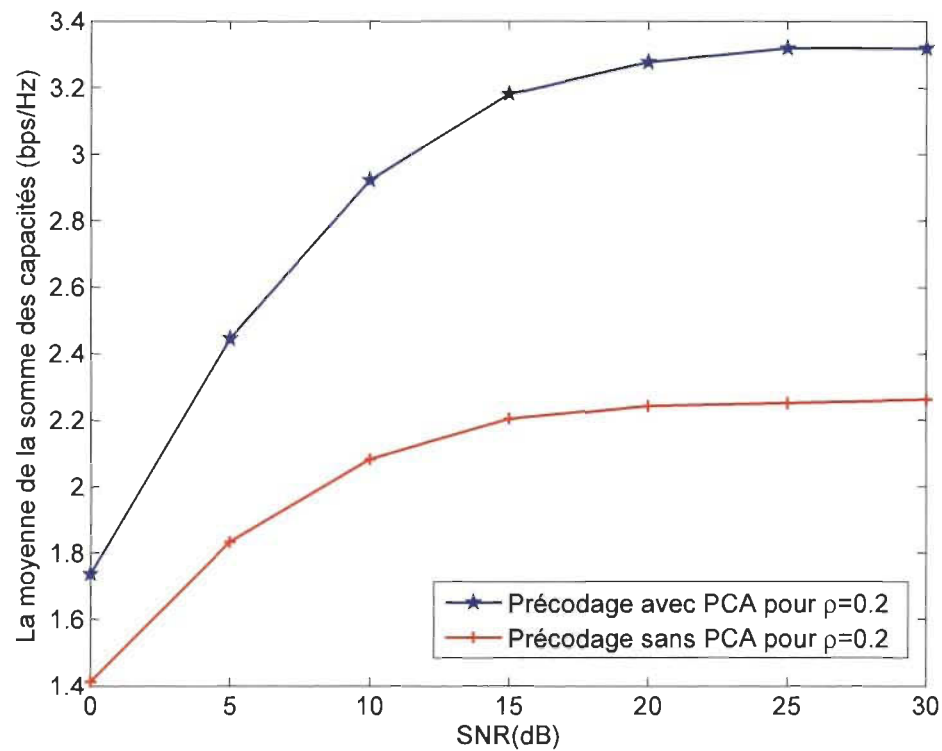
Figure 6.3. Comparaison de la moyenne de la somme des capacités entre le précodage avec et sans PCA pour un système MU-MIMO avec K = 2 , N_t = 2 , N_r = 2 et B = 4 bits, sous un canal corrélé avec un faible niveau de corrélation spatiale, \rho = 0.2 .
