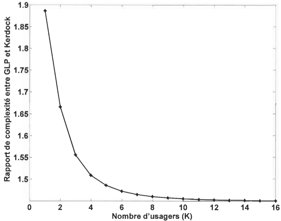
Figure 3.6. Rapport de complexité entre le précodage à base des codebooks GLP et de Kerdock.
