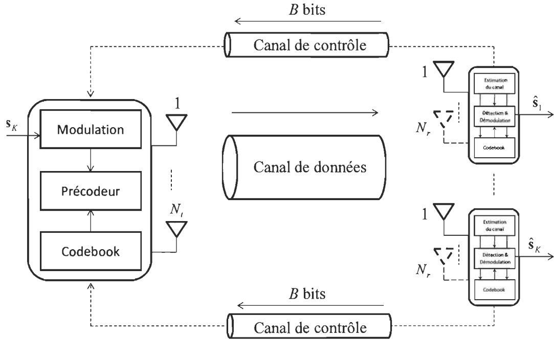
Figure 2.2. Système MIMO multi-utilisateur avec précodage unitaire.
