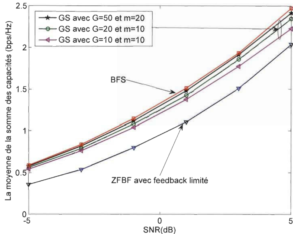
Figure 5.9. Comparaison de la moyenne de la somme des capacités entre le BFS, le ZFBF avec feedback limité [8] et le GS avec ( m = 10, G = 20 ; m = 20, G = 50 et m = 50, G = 100 ) pour un système MU-MIMO avec K = 2 , N_t = 2 , N_r = 1 et B = 8 bits.
