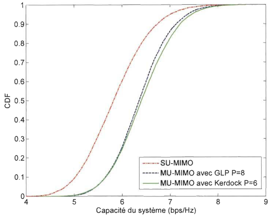
Figure 3.3. La CDF de la capacité des systèmes SU-MIMO et MU-MIMO avec parfaite CSIT pour X = 10 , K = 2 , N_t = 2 et N_r = 2 .
