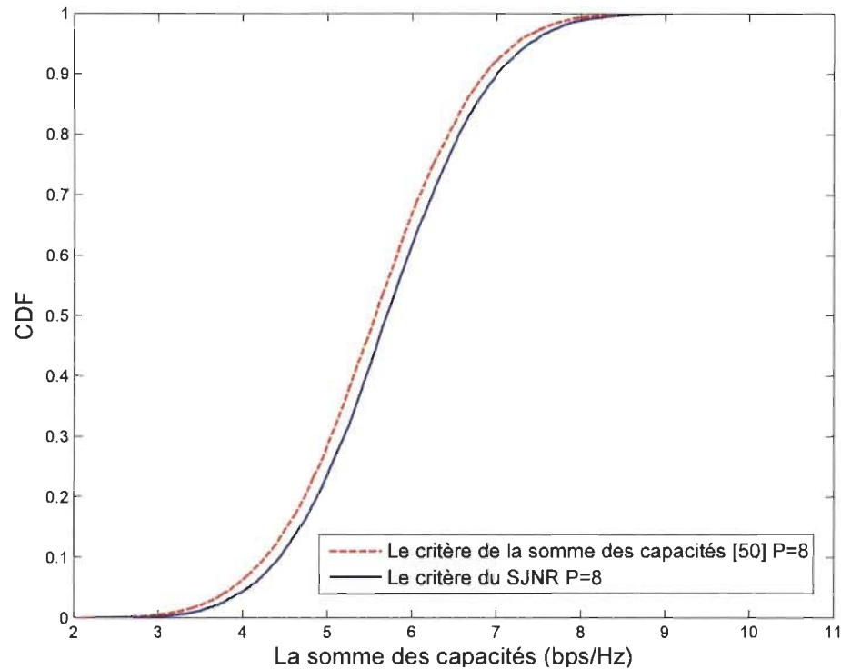
Figure 4.3. Comparaison de la CDF de la somme des capacités entre le critère de la maximisation du SJNR et le critère de Fang et al. [50] pour un système MU-MIMO avec K = 2 , N_t = 2 et N_r = 2 .
