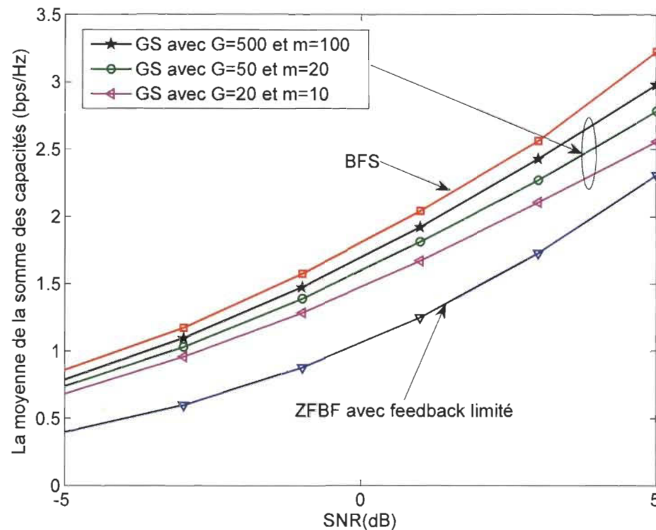
Figure 5.10. Comparaison de la moyenne de la somme des capacités entre le BFS, le ZFBF avec feedback limité [8] et le GS avec ( m = 10, G = 20 ; m = 20, G = 50 et m = 50, G = 100 ) pour un système MU-MIMO avec K = 3, N_t = 3, N_r = 1 et B = 8 bits.
