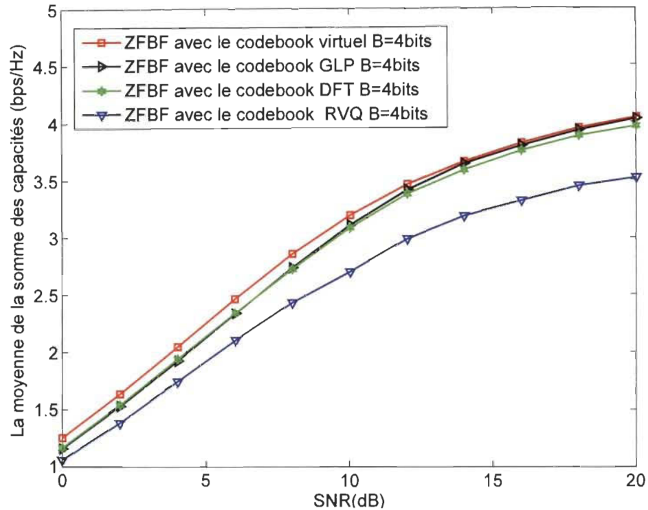
Figure 3.13. Comparaison en termes de moyenne de la somme des capacités entre le codebook virtuel avec b = 1 et les codebooks RVQ, GLP et DFT pour un système MU-MIMO avec N_t = 4 et B = 4 bits.
