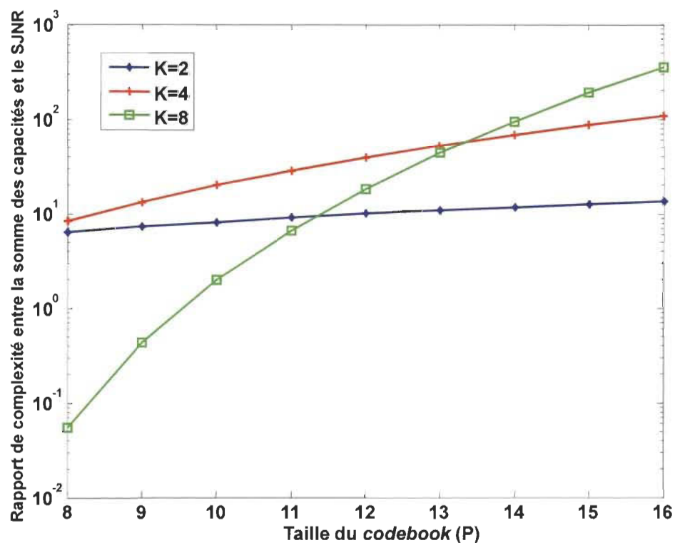
Figure 4.5. Rapport de complexité entre le critère de la maximisation du SJNR et le critère de Fang et al. [50] en fonction de la taille du codebook (P).
