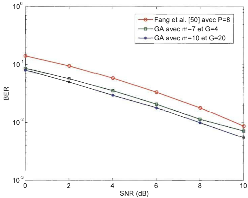
Figure 4.9. Comparaison en BER entre le précodage à base de GA et la méthode de Fang et al. [50] pour un système MU-MIMO avec K = 2 , N_t = 2 et N_r = 2 .
