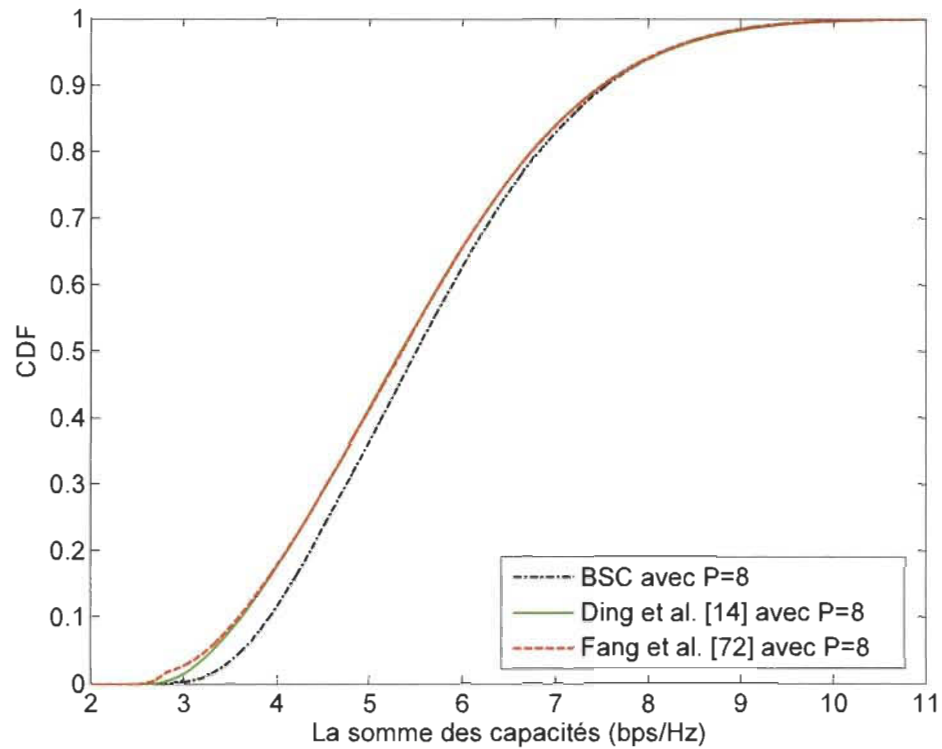
Figure 5.2. Comparaison de la CDF de la somme des capacités entre le BSC, la méthode de Fang et al. [72] et la méthode de Ding et al. [14] pour un système MU-MIMO avec K = 2 , N_t = 2 , N_r = 2 et B = 4 bits.
