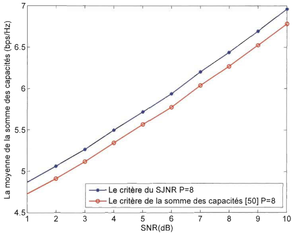
Figure 4.4. Comparaison de la moyenne de la somme des capacités entre le critère de la maximisation du SJNR et le critère de Fang et al. [50] pour un système MU-MIMO avec K = 2 , N_t = 2 et N_r = 2 .
