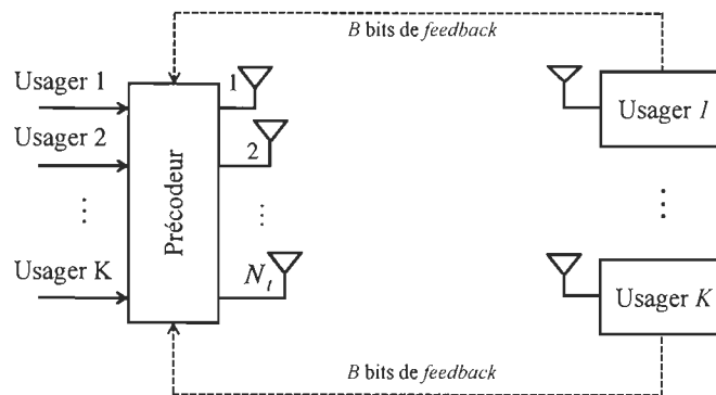
Figure 3.8. Schéma synoptique d'un système MU-MIMO avec une seule antenne dans chaque récepteur.
