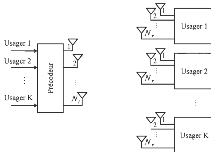
Figure 2.1. Système MIMO multi-utilisateur en liaison descendante.
