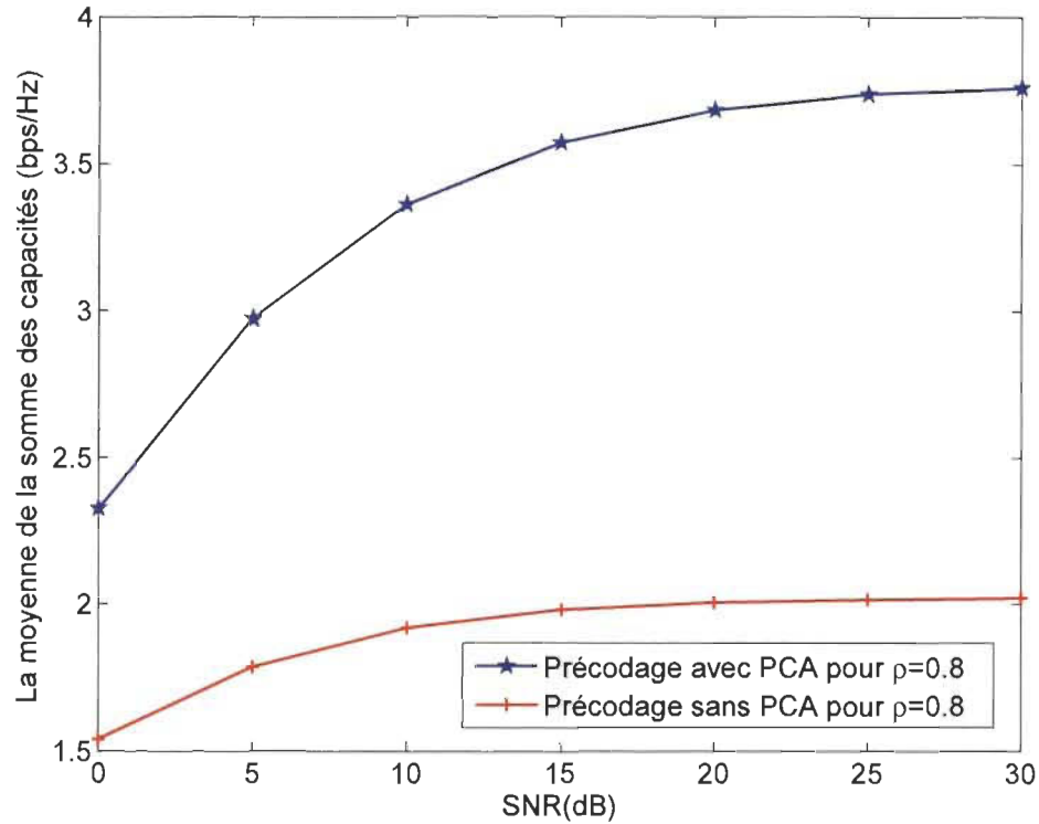
Figure 6.4. Comparaison de la moyenne de la somme des capacités entre le précodage avec et sans PCA pour un système MU-MIMO avec K = 2 , N_t = 2 , N_r = 2 et B = 4 bits, sous un canal corrélé avec un fort niveau de corrélation spatiale, \rho = 0.8 .
