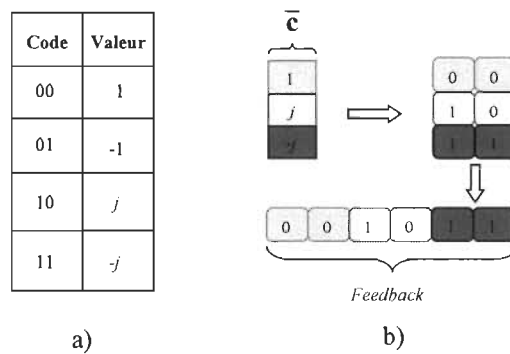
Figure 3.7. (a) Codage des éléments du codeword et (b) Conversion du codeword en bits de feedback lorsque N_t = 3 et b = 2 .
