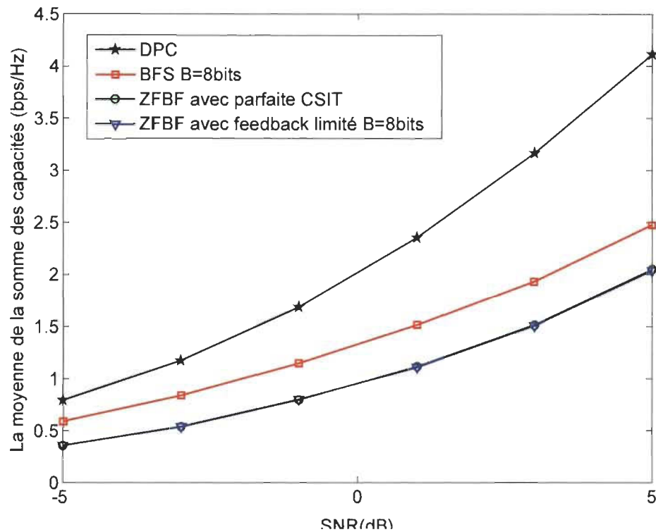
Figure 5.4. Comparaison de la moyenne de la somme des capacités entre le DPC, le BFS, le ZFBF avec parfaite CSIT et feedback limité [8] pour un système MU-MIMO avec K = 2 , N_t = 2 , N_r = 1 et B = 8 bits.
