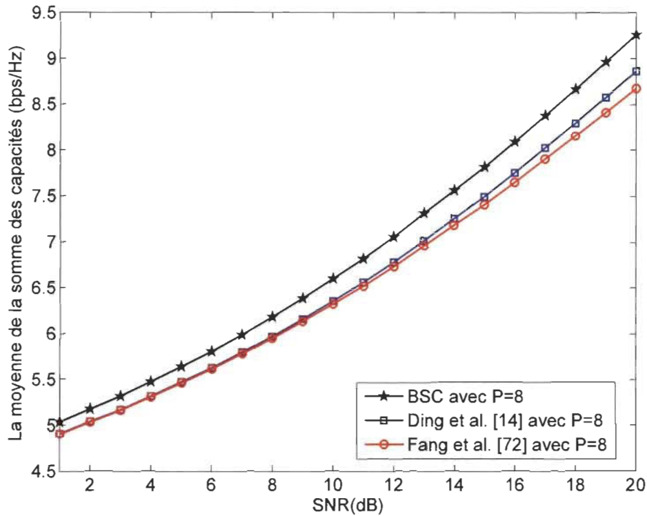
Figure 5.3. Comparaison de la moyenne de la somme des capacités entre le BSC, la méthode de Fang et al. [72] et la méthode de Ding et al. [14] pour un système MU-MIMO avec K = 2 , N_t = 2 , N_r = 2 et B = 4 bits.
