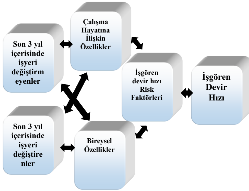
Şekil 1: Araştırma Modeli
