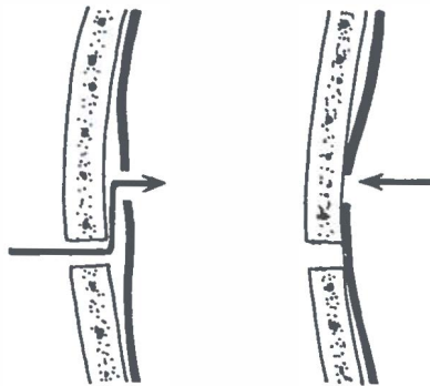
fig. 13. ventielmechanisme.
