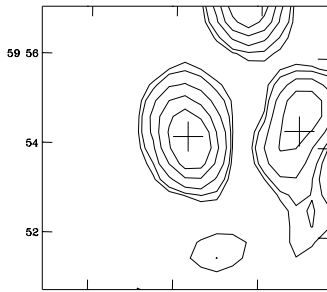
WNB1748+5954 S
