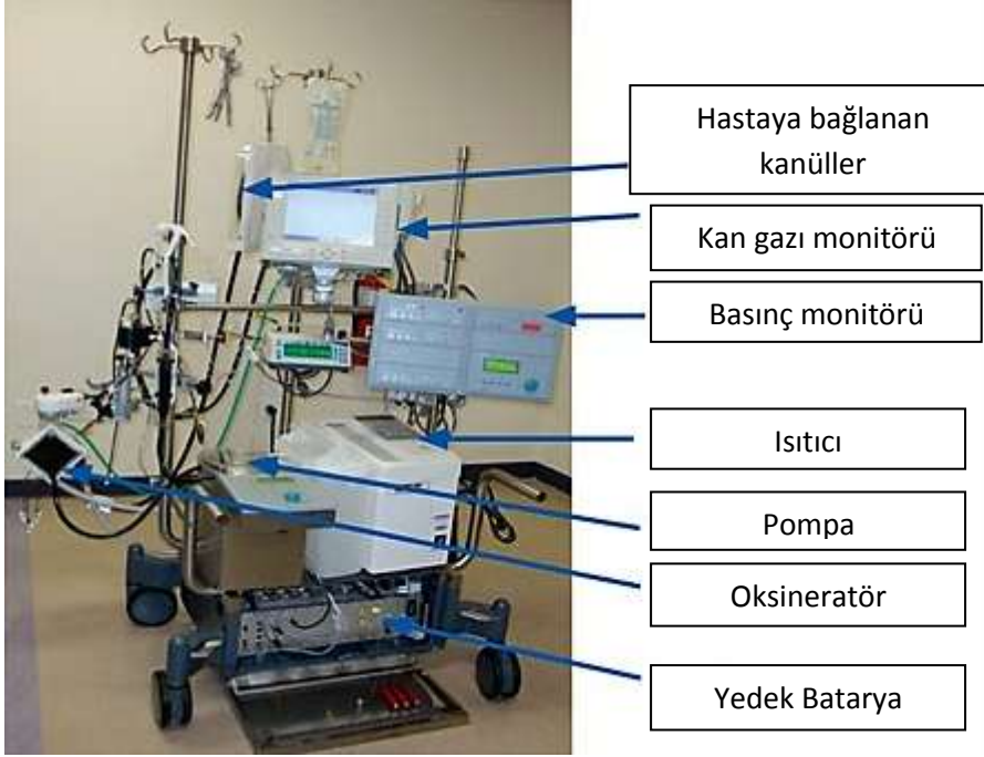
Şekil 2.1. ECMO sistemi
