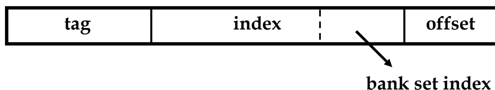
Figura 3.2 - Indirizzo fisico di una cache D-NUCA
