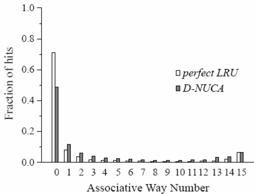
Figura 1.8 - Distribuzione delle hit per LRU e generational promotion
