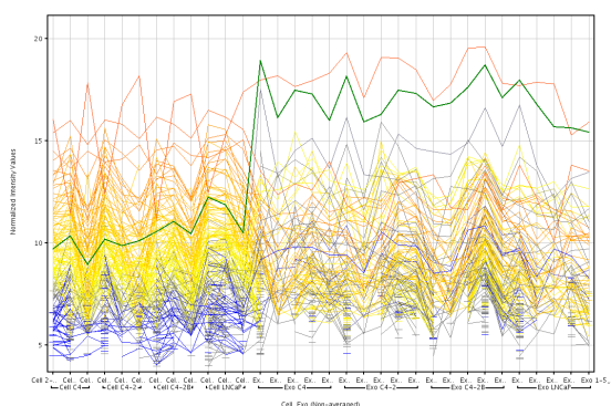
図 1. ヒト前立腺癌細胞株の細胞内およびエクソソーム中の miRNA の発現プロファイル
