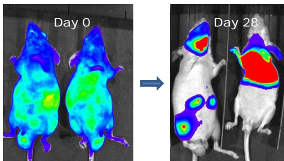
図 4. 癌転移の in vivo imaging
