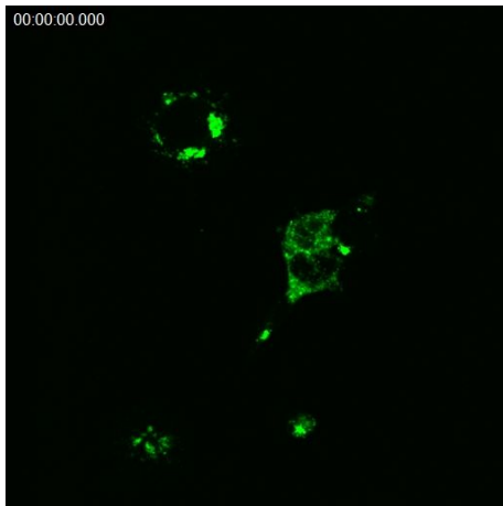
図 3. エクソソームを取り込んだ細胞
