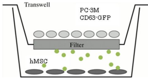
図 2. Transwell 培養モデル
