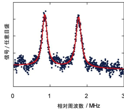
図1 太いビームと結合する光共振器セルを使った \text{CH}_3\text{D} の飽和吸収スペクトル
