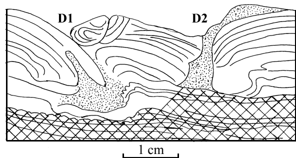
Fig. 2 – dessin de lame mince. D1 et D2 : traces de doigts. En blanc : sédiments algolaminés, avec matérialisation des laminations planes, onduleuses ou très déformées. Pointillés : micrite claire. Croisillons : zone indurée précocement ayant résisté au poids des animaux. Dessin d'après FREYTET, in DEMATHIEU et al. , 2000, fig. 61, redessiné et réinterprété.
