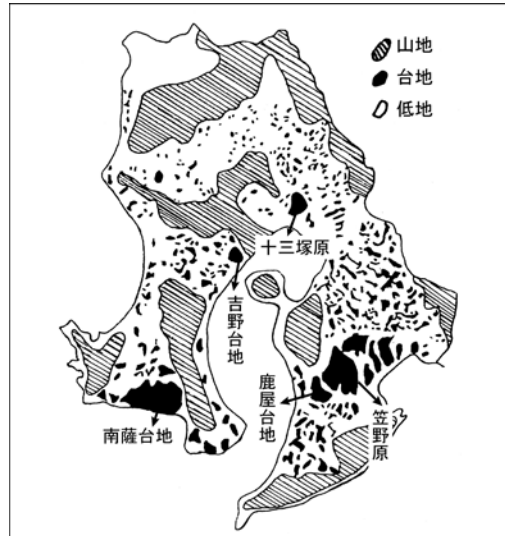
図 15. 鹿児島県のシラス分布(佐野, 1997 を一部改変)。
