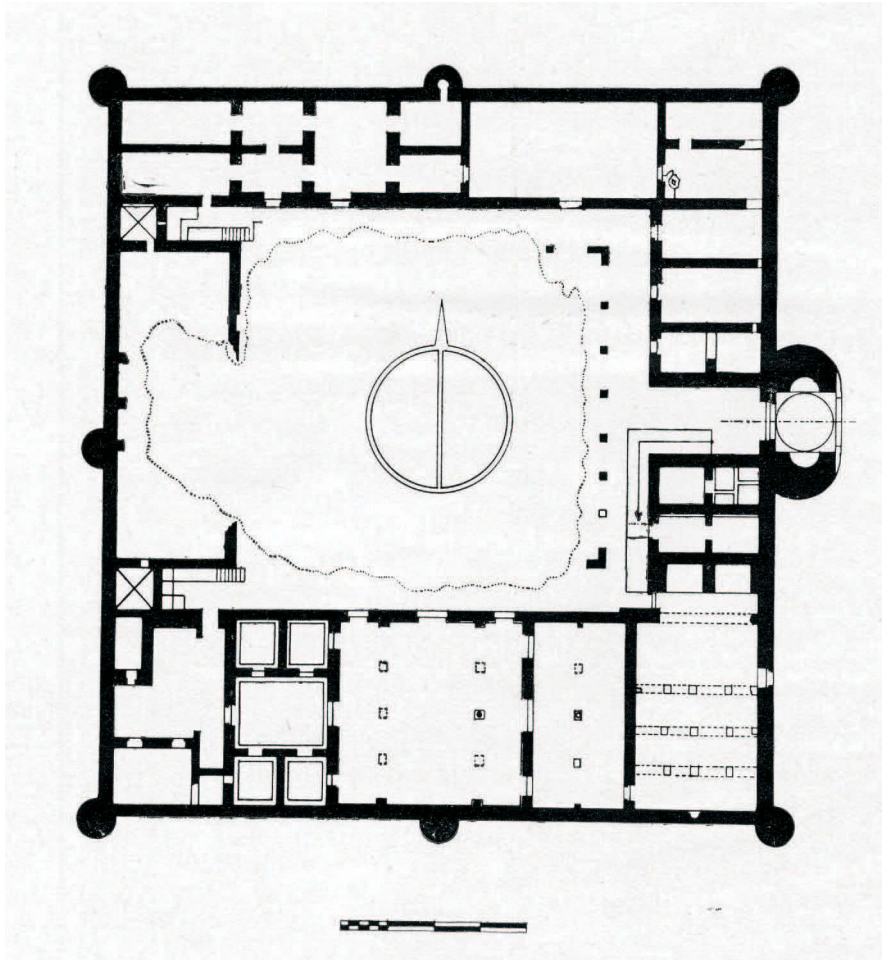
Abb. 16, oben: Endgültige Rekonstruktion von Minya nach der letzten Ausgrabungskampagne 1938/39. Abb. 17, unten: Luftbildaufnahme der Anlage durch Oberleutnant Holt der britischen Militärbesatzung in Tiberias. (Puttrich-Reignard 1939, Lageplan und Abb. 1)
