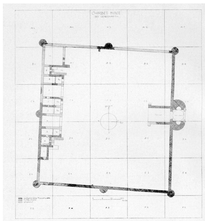
Abb. 8: Minya nach den Ausgrabungen Schneiders 1936, Rekonstruktion. (Schneider & Puttrich-Reignard, Ein frühislamischer Bau am See Genezareth, Fig. 5)
