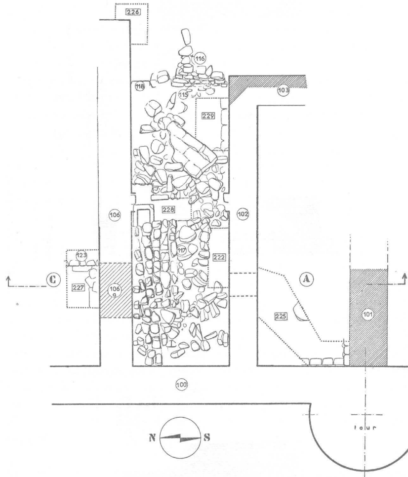
Abb. 20, oben: Die Räume A-B-C mit Suchschnitten. Abb. 21, unten: Querschnitt durch A-B-C, ermittelt durch 225-222-227. (Grabar 1960, S. 231, Fig. 5 und S. 232, Fig. 6).
