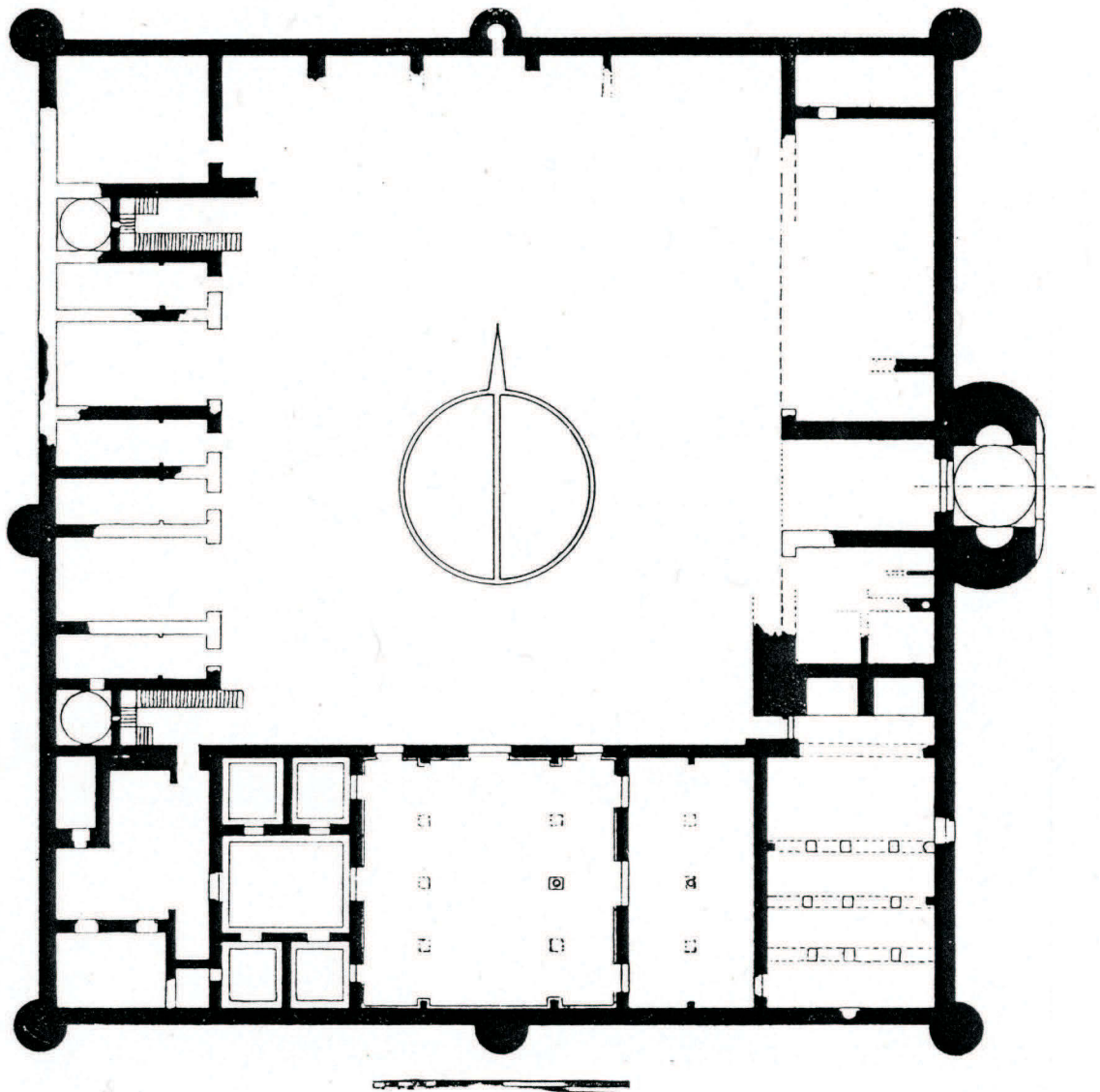
Abb. 15: Grundriss von Minya nach der Herbstkampagne unter Leitung von Puttrich-Reignard 1937/38 (Puttrich-Reignard 1938, in: Berliner Museen, S. 81, Abb.1)
