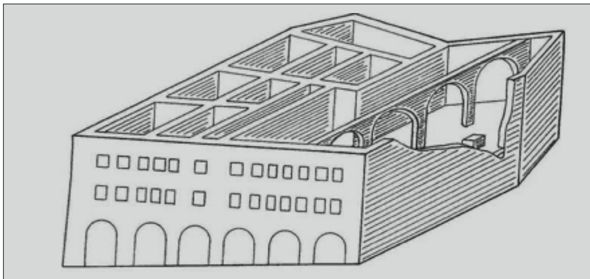
Fig. 1a. Roma: ricostruzione del complesso abitativo con utilizzazione culturale cristiana su cui si impiantò la chiesa dei SS. Giovanni e Paolo al Celio (da Krautheimer 1937)
