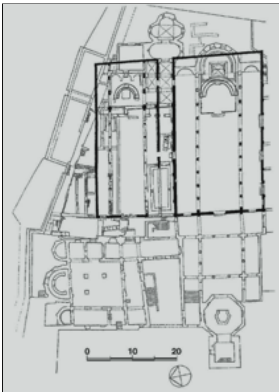
Fig. 16. Parenzo: schema ricostruttivo della basilica doppia preeufrasi-ana (metà del sec. V) (da Matejčić, Chevalier 1998)
