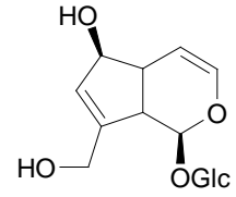
6 aucubin
