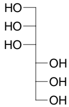
1 mannitol
