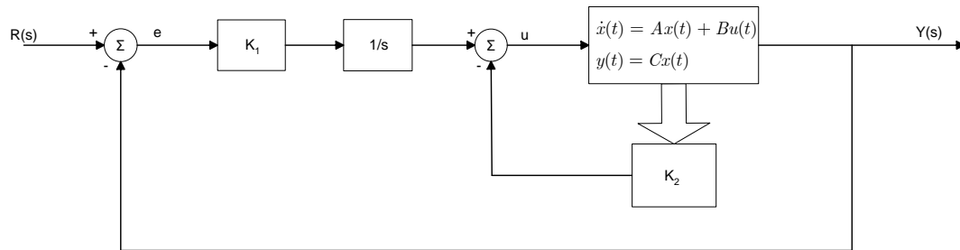
Σχήμα 1: Διάγραμμα μοντέλου εσωτερικού ελέγχου
