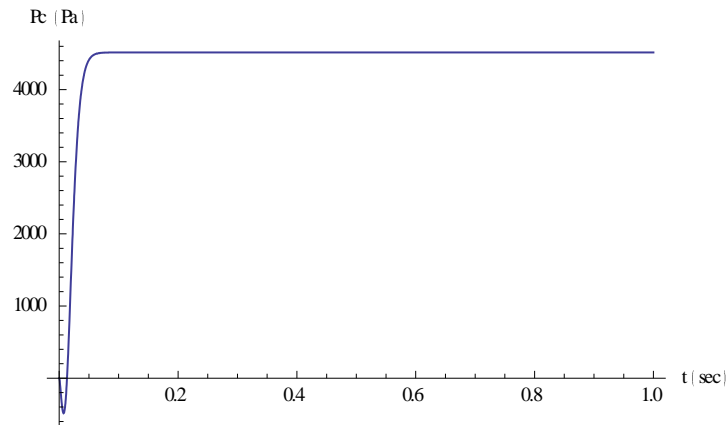
Εικόνα 5.6: Πίεση εντός θαλάμου αντλίας
