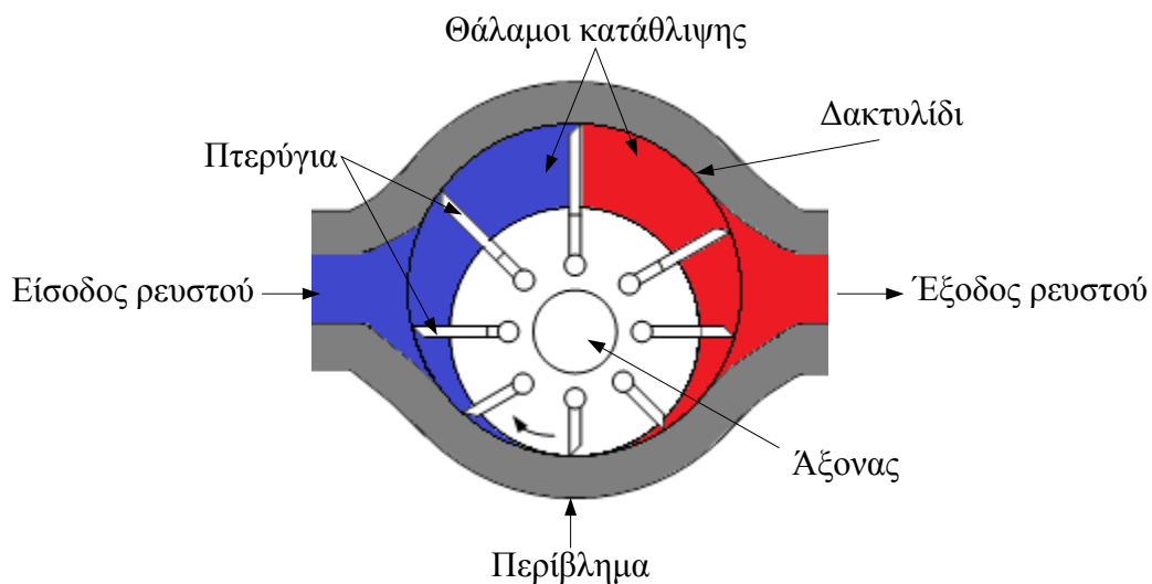
Εικόνα 2.7: Πτερυγιοφόρα αντλία – μη ισορροπημένη
