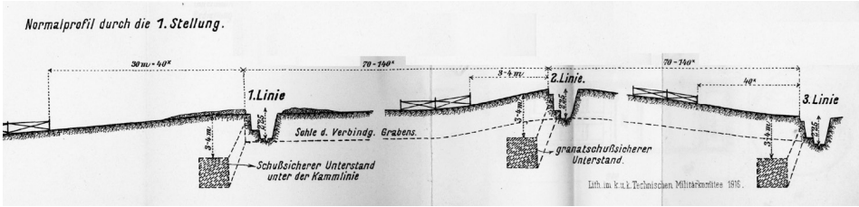
Abb.2 Vorschrift 1915 – Normalprofil: Seitenquerschnitt der so genannten ›1. Stellung‹, bestehend aus drei Linien. Quelle: Anhaltspunkte 1915.
