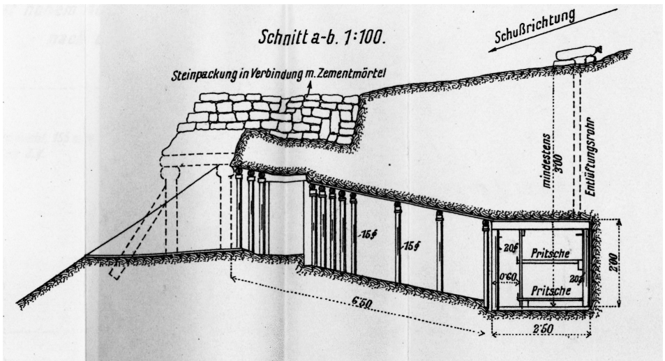
Abb. 3 Unterschiedliche Ausführungen von Unterständen für Stellungsinfanterie ab dem Jahre 1915. Quelle: Anhaltspunkte 1915.
