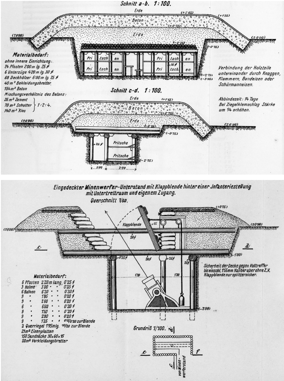
Abb.4 Unterschiedliche Ausführungen von Unterständen für Stellungsinfanterie ab dem Jahre 1915.
