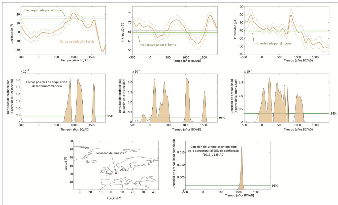
Fig. 8. Datación arqueomagnética de horno en Bélgica. En la parte superior se muestra las curvas patrones para la declinación, inclinación e intensidad con su error al 95% (curvas naranjas). Además se muestra el dato que se va a datar con su error (líneas verdes). En el panel central se indican las diferentes funciones de probabilidad de cada elemento geomagnético. Y en la parte inferior un mapa con la localización del sitio arqueológico y la datación final. Se recomienda consultar la versión digital.
