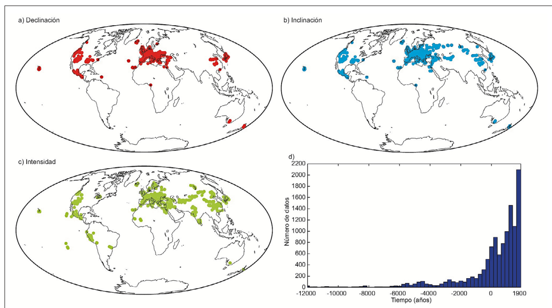
Fig. 4. Distribución mundial de datos arqueomagnéticos para los últimos 14 milenios. a-c) Mapa con los datos direccionales y de intensidad, d) Distribución temporal de los datos direccionales y de intensidad (todos los datos conjuntos).
