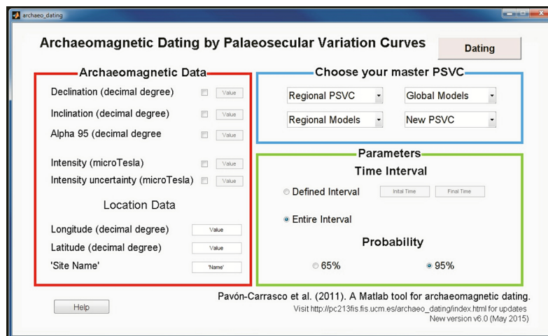
Fig. 7. Programa de datación arqueomagnética. Se muestra la ventana interactiva del programa de datación arqueomagnética archaeo_dating que se usa para la práctica.
