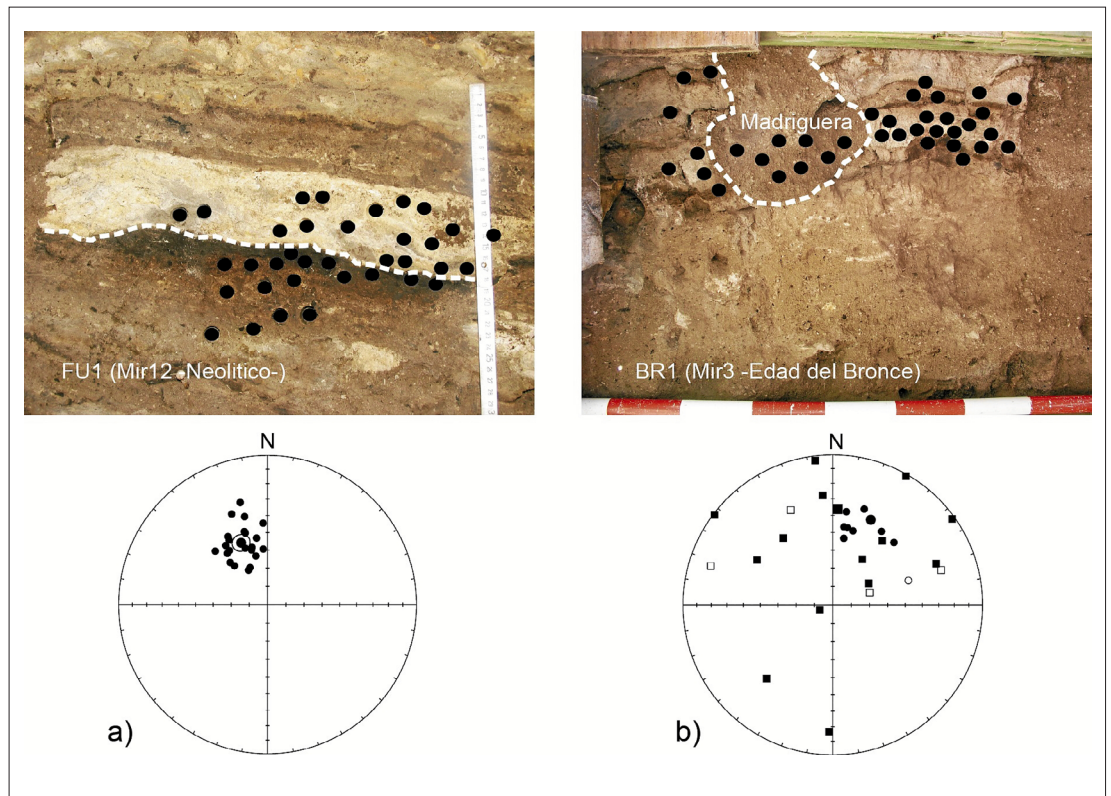
Fig. 6. Estudio direccional en dos episodios de combustión de la cueva de El Mirador (Burgos). (a) Episodio neolítico bien conservado. (b) Episodio alterado por una madriguera. Abajo sus correspondientes estereogramas con las direcciones arqueomagnéticas medias de las muestras estudiadas. Los círculos en la figura 6b representan las muestras quemadas no bioturbadas y los cuadrados, las muestras de dentro o anexas a la madriguera y que sí han sufrido bioturbación (no in situ ). Modificado de Carrancho et al. (2012).
