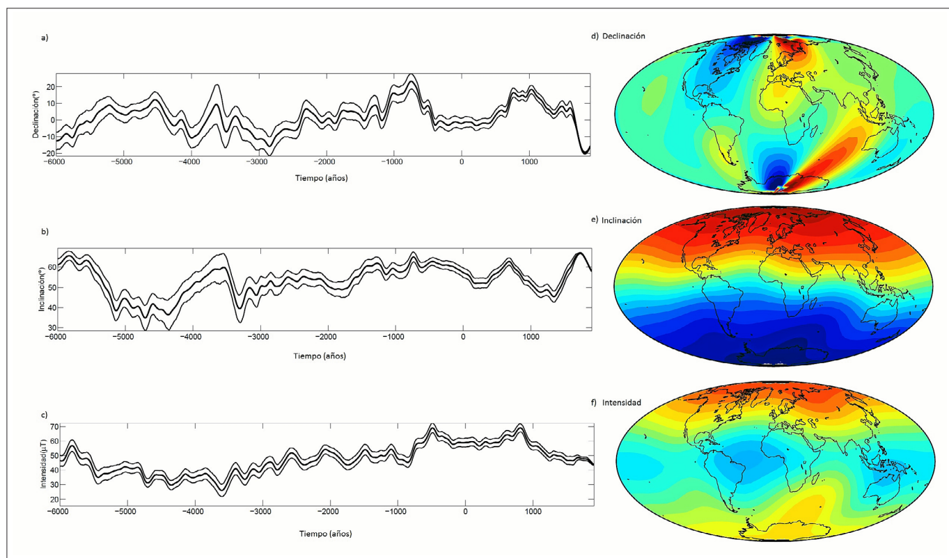
Fig. 5. Variación del campo geomagnético en el pasado. a-c) Curva de variación secular del campo magnético de la Tierra en Madrid para los últimos 8000 años. d-f) Mapas de los elementos geomagnéticos para el año 1200 d.C. dados por el modelo global arqueomagnético SHA.DIF.14k (Pavón-Carrasco et al. , 2014).
