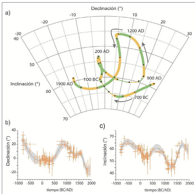
Fig. 3. Curva de variación secular (direccional) para Iberia. Obtenida a partir del estudio de materiales arqueológicos quemados de cronología bien definida. Figura modificada de Gómez-Paccard et al. (2006b).
