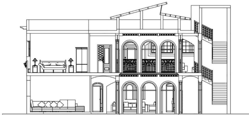
قطاع B-B مقياس الرسم 1:100
