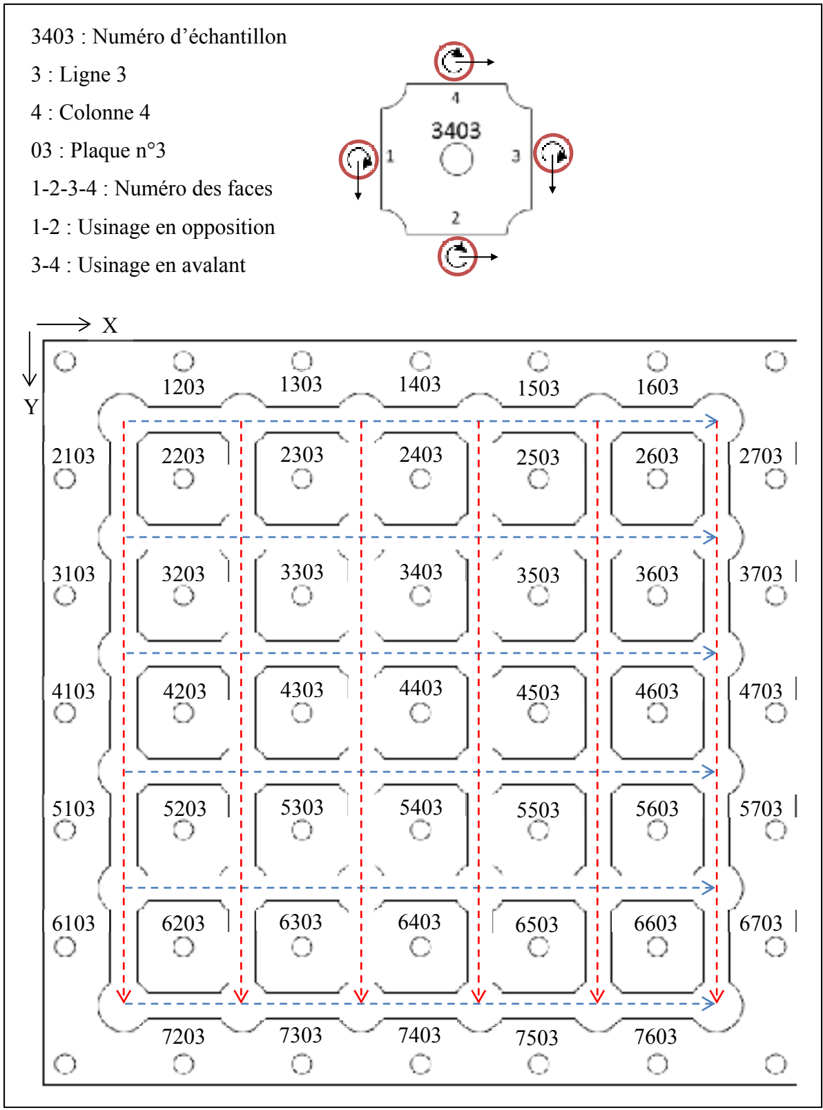
Figure 2.39 : Nomenclature et opérations exécutées sur la plaque #3
