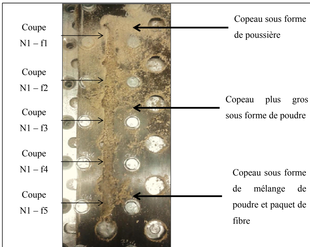
Figure 2.43 : Aspect du copeau en fonction de la vitesse d'avance pour les fibres orientées à 0^\circ
