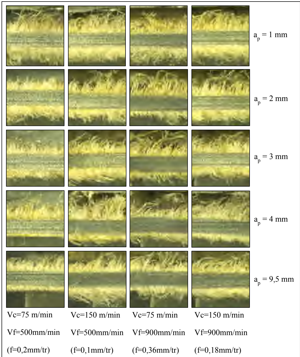
Figure 2.28 : Sections usinées en opposition avec l'outil revêtu diamant CVD en fonction des différents paramètres de coupe
