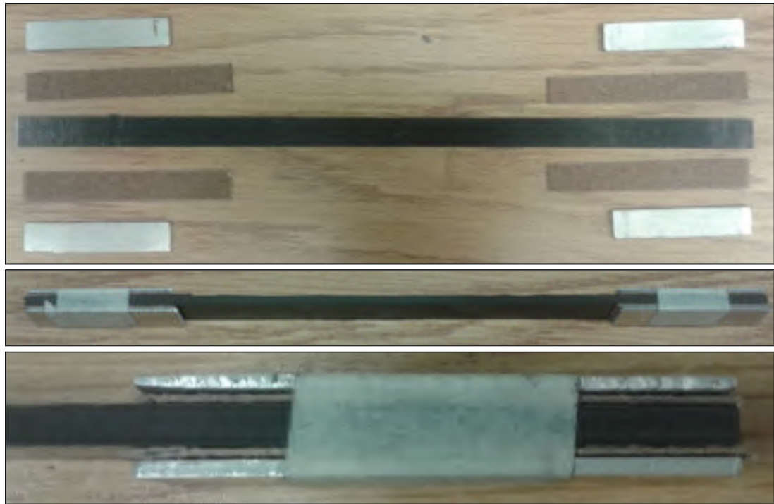
Figure 1.24 : Éprouvette de traction
