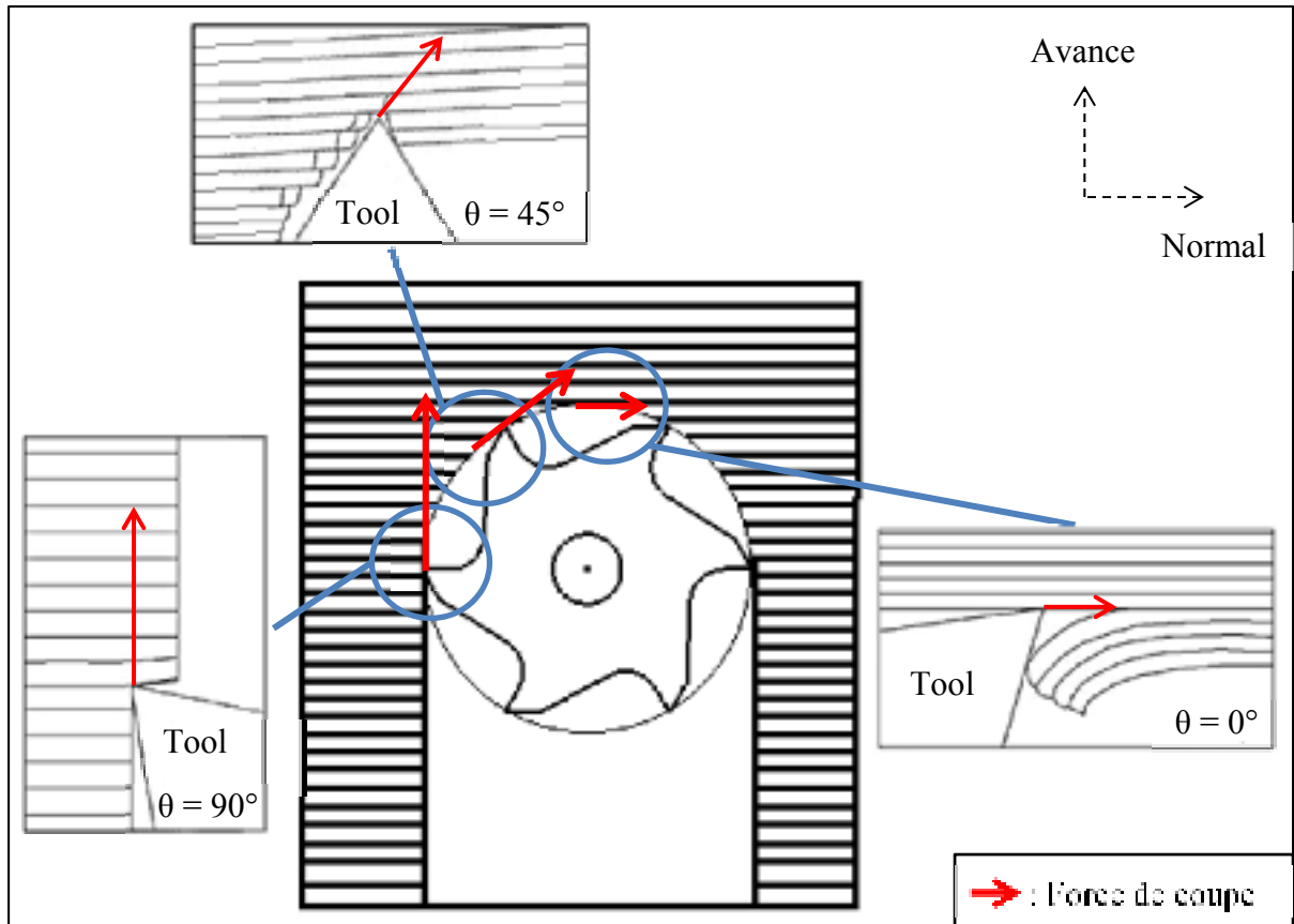
Figure 2.69 : Schéma d'usinage suivant pour l'orientation des fibres à 90^\circ avec plein engagement de l'outil
