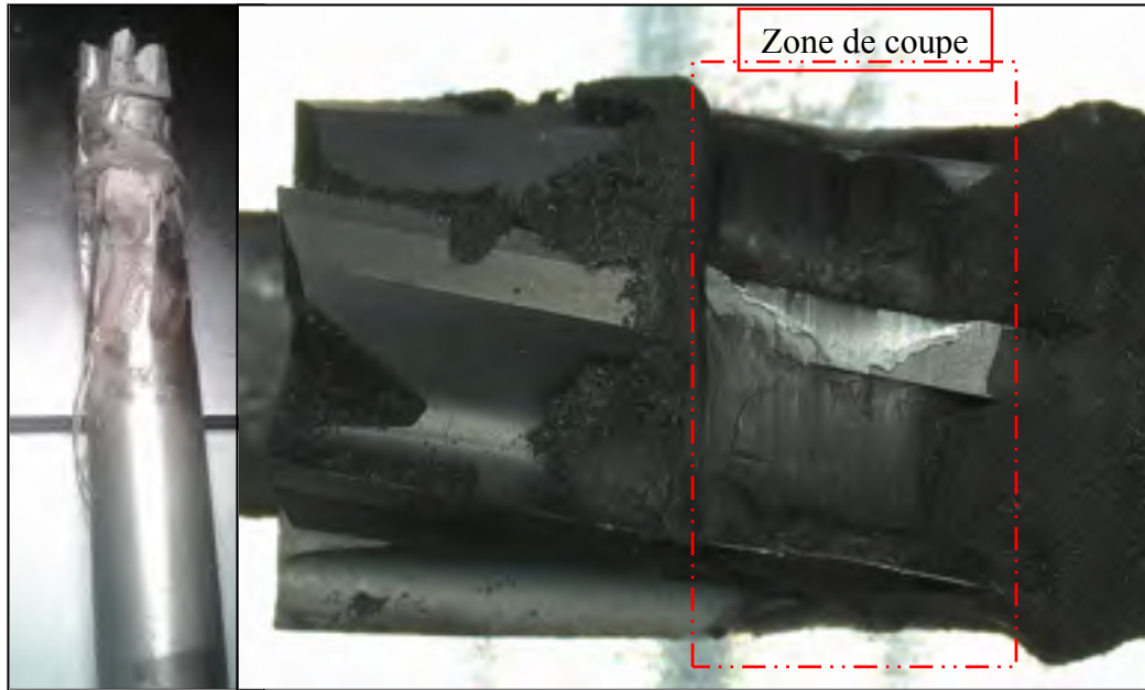
Figure 1.30 : Zone de coupe après usinage (outil usé)
