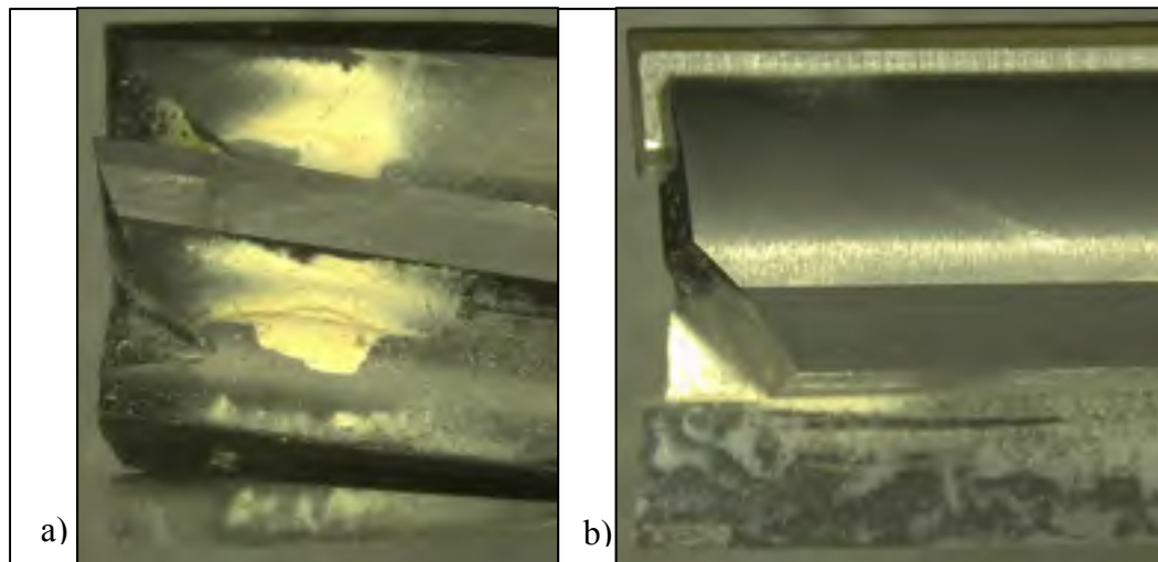
Figure 2.44 : Outil après 3.12 m de coupe, a) outil 6 lèvres (outil #1), b) outil 2 lèvres (outil #2) - Usure nulle
