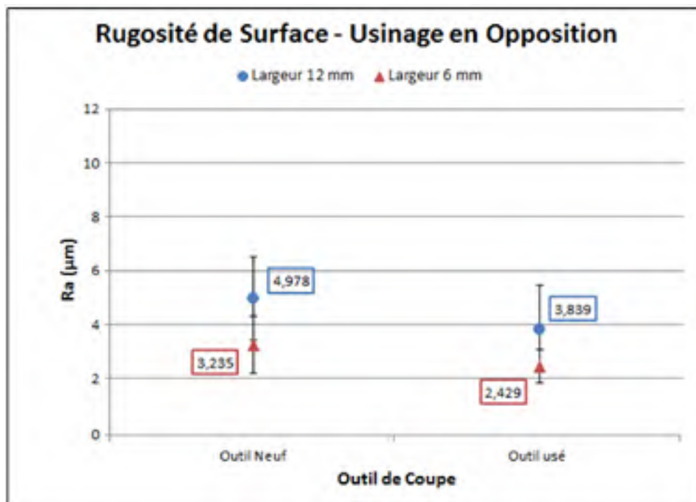
Figure 1.36 : Rugosité longitudinale du pli à -45^\circ pour le mode en opposition
