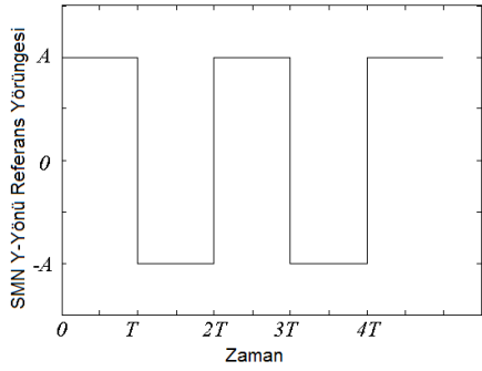
Şekil4: Yumuşatma öncesi SMN y-yönü referansı.
