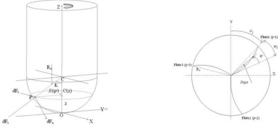
Şekil 1. Küresel uçlu freze geometrisi
