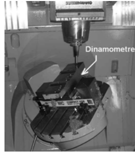
Şekil 7. Deney Düzeneği
