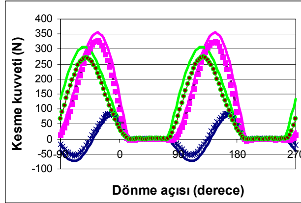
Şekil 8 . Benzetimi Yapılan ve Ölçülen Kesme Kuvvetleri Karşılaştırması
