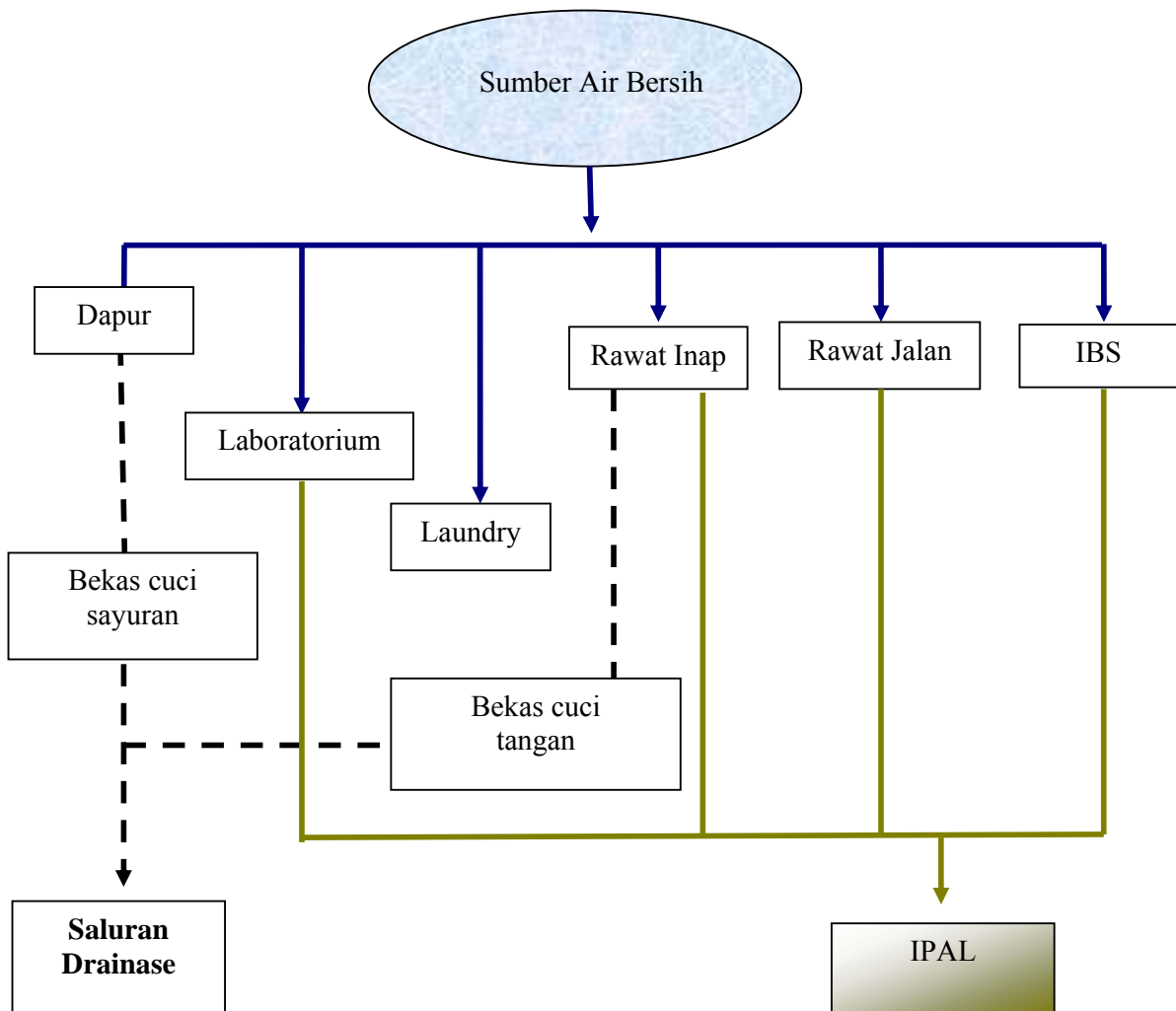
Gambar 4.9. Diagram Alir Pengelolaan Air Bersih Rumah Sakit Umum Daerah Ungaran
