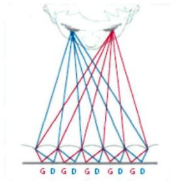
Figure 29. Diagramme montrant un système à réseau lenticulaire.
