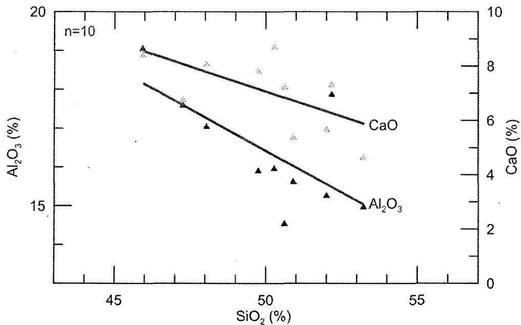
Figure 2.14. Diagramme montrant la corrélation entre l'enrichissement en silice et l'appauvrissement en \text{Al}_2\text{O}_3 (triangles noirs) et \text{CaO} (triangles gris) pour les laves mafiques du Membre de Sordide.
