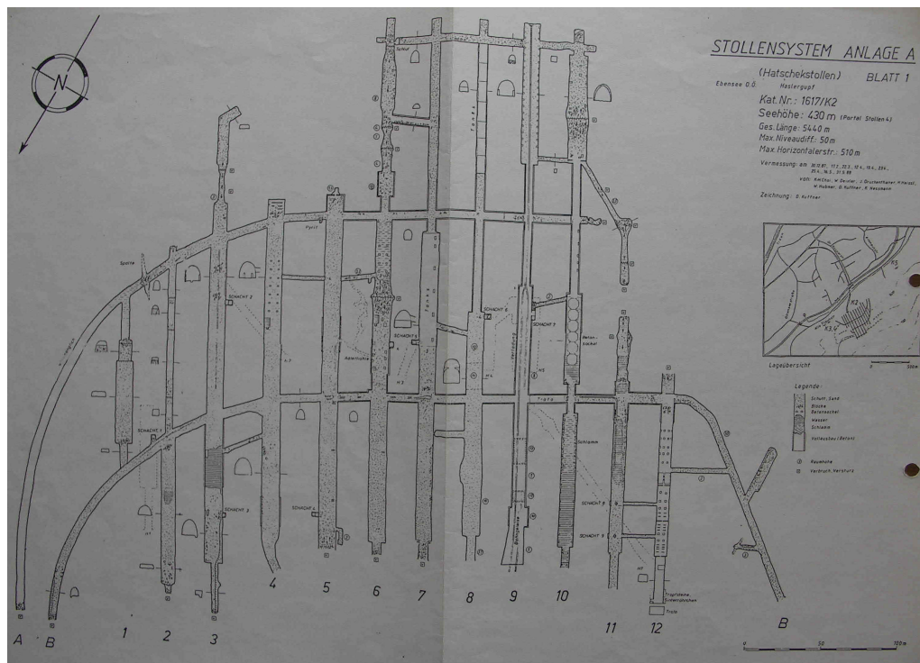
Bild 5: Stollensystem Anlage A. Gesamtlänge 5440m.
